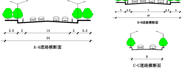
道路横断面（单位：m）
