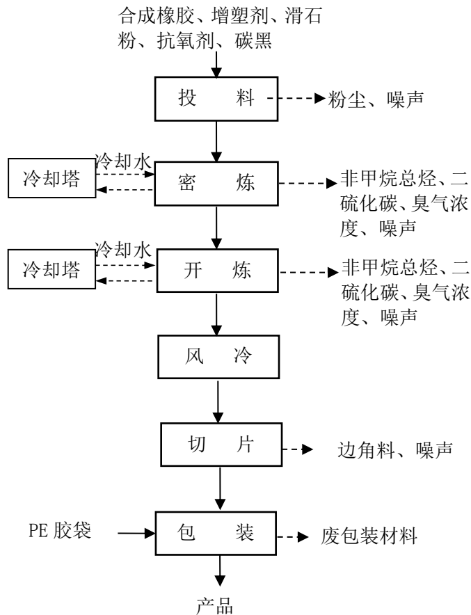
图 2-2 项目橡胶胶片生产工艺流程图
