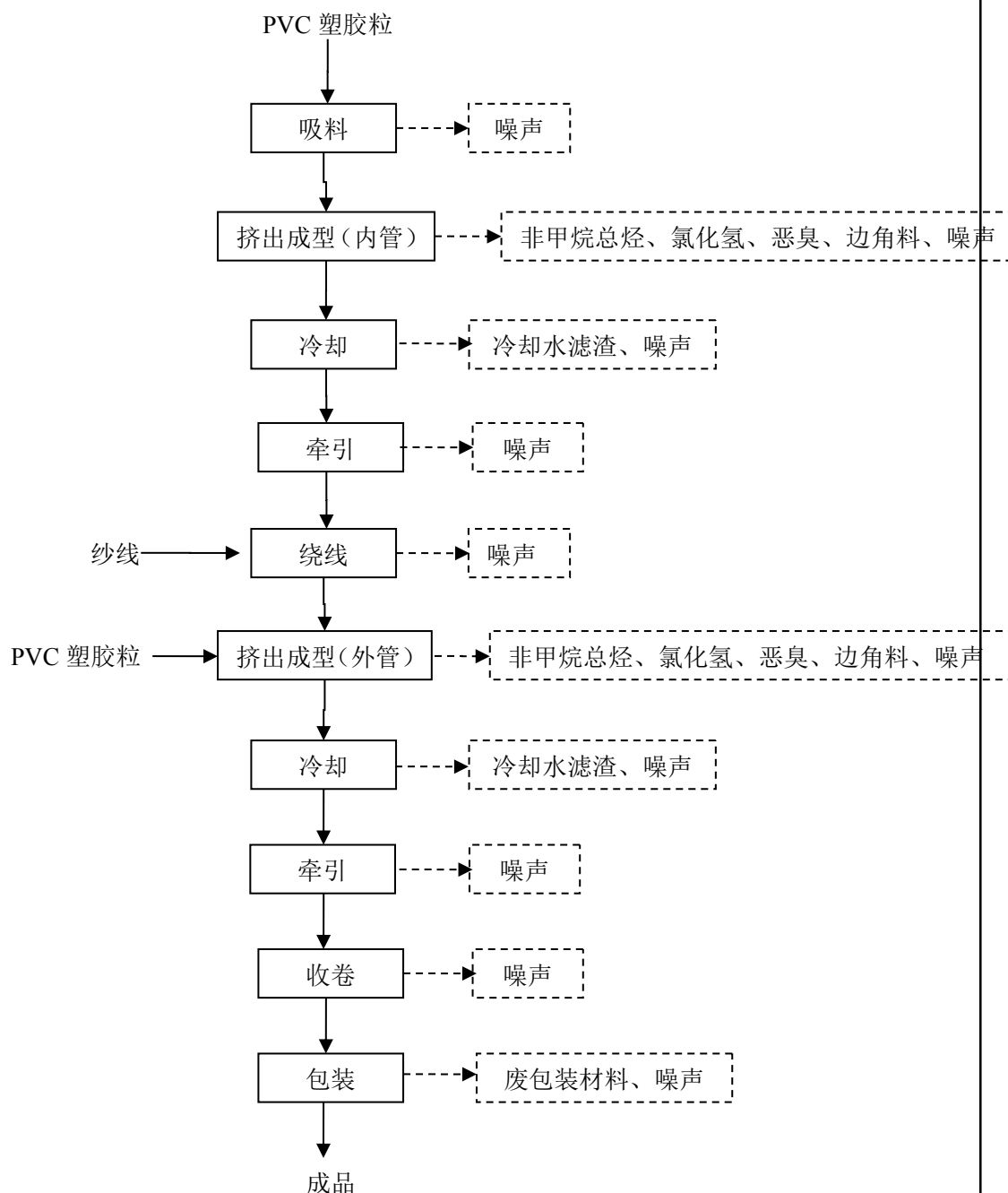
图 2-3 PVC 软管生产工艺流程及产污节点图
