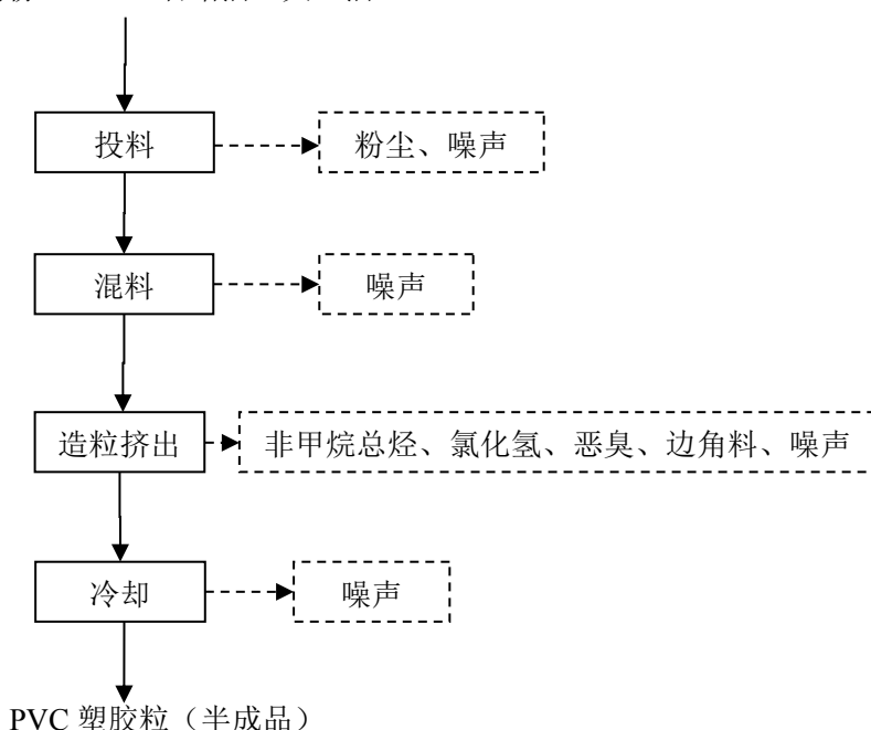
图 2-2 PVC 塑胶粒（半成品）生产工艺流程及产污节点图
