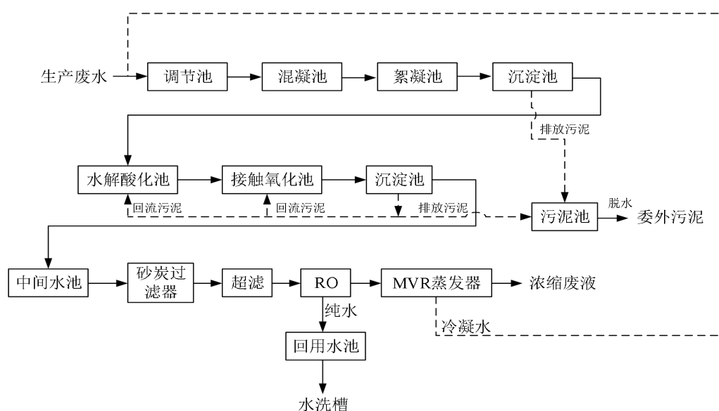
图6 项目生产废水处理工艺流程图
