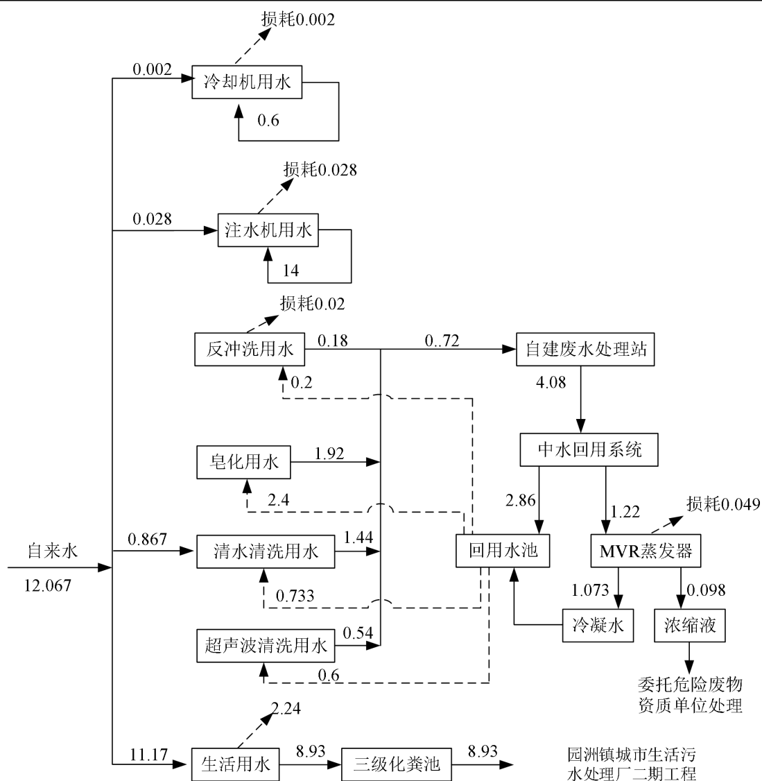
图 1 项目最大日水量平衡图（单位：t/d）
