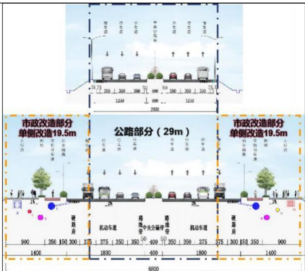
图2-3 上园路标准段(4.104km)两侧各改造19.5m横断面图
