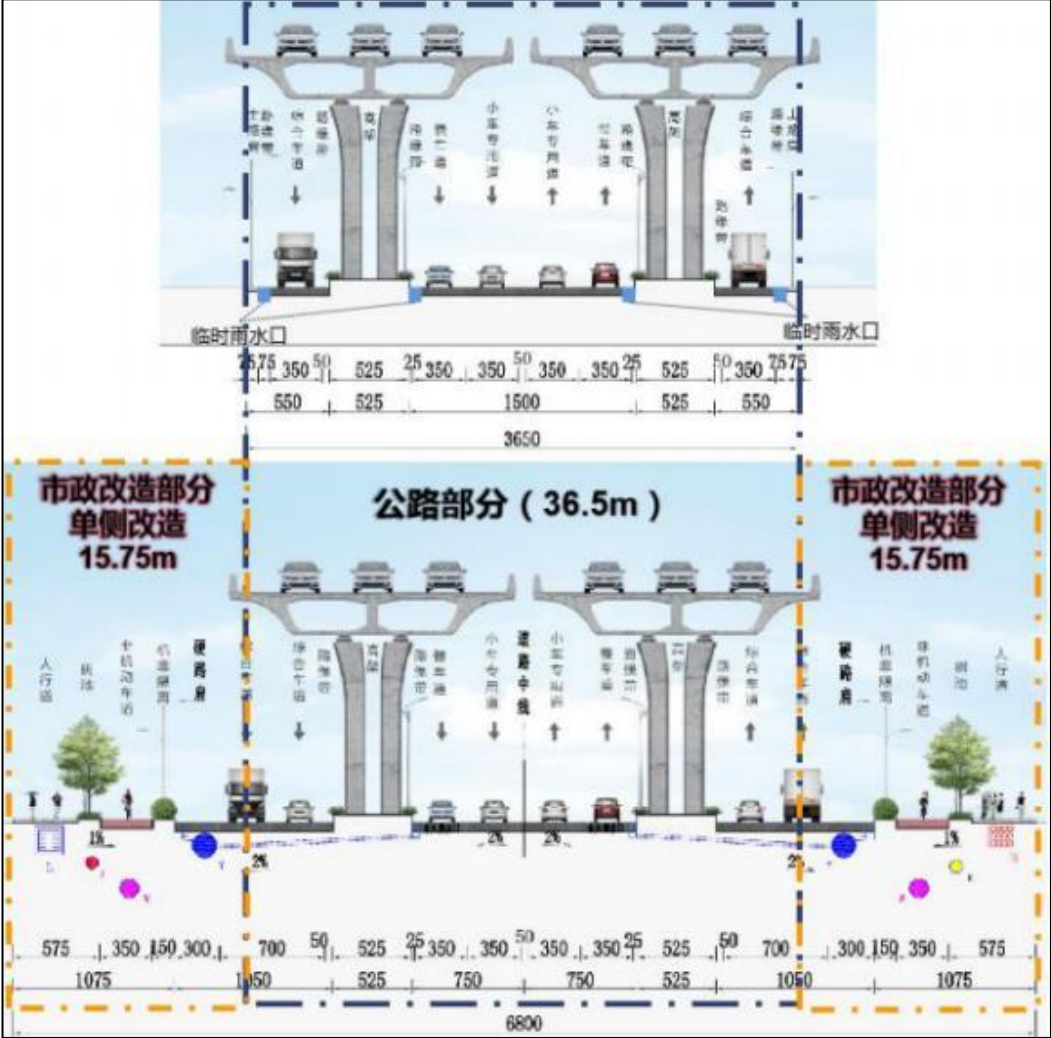
图2-2 上园路与从莞高速共走廊段(2.12km)两侧各改造15.75m横断面图
