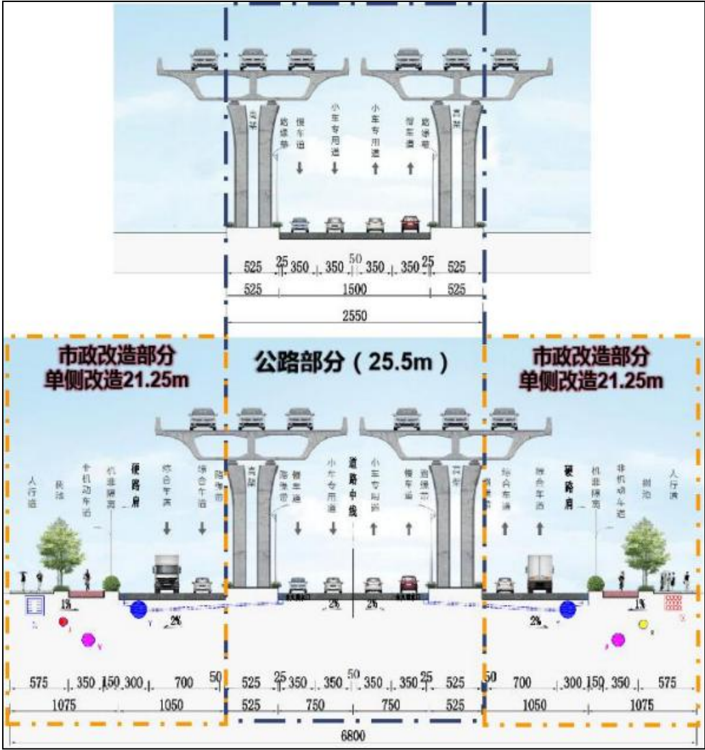
图2-1 东坡大道欣旺达片区段 (1.22km ) 两侧各改造 21.25m横断面图
