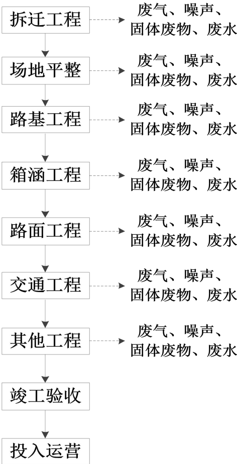
图 2-10 项目道路工程施工工艺流程及产污环节图
