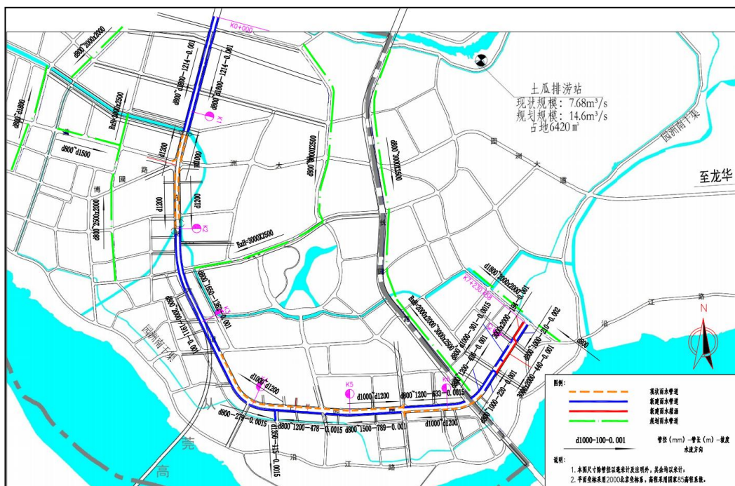
图 2-6 雨水管道总平面布置图
