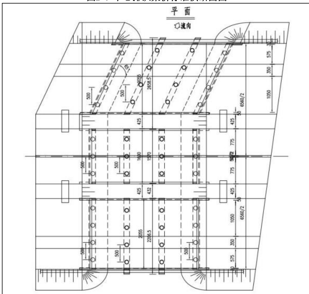
图 2-5 中心排洪渠桥标准平面图
