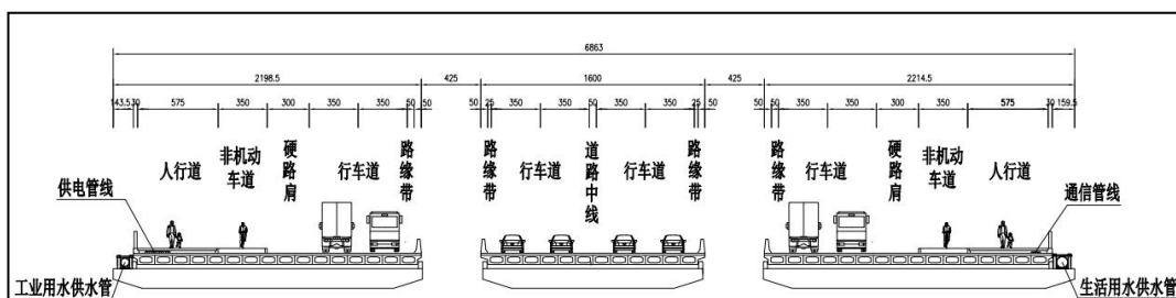
图2-4 中心排洪渠桥标准横断面图
