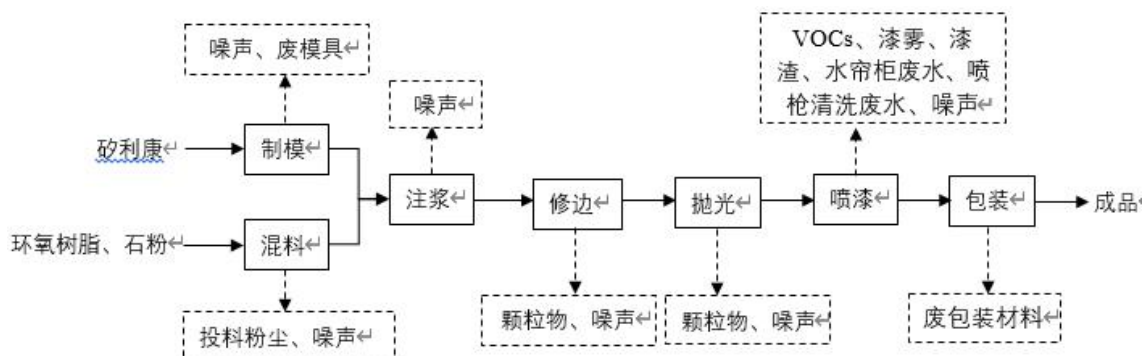
图 2.6-1 工艺品摆件生产工艺流程及产污节点图
