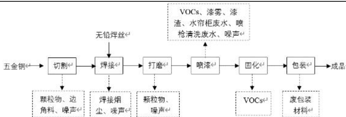
图 2.6-2 五金铜工艺品生产工艺流程及产污节点图
