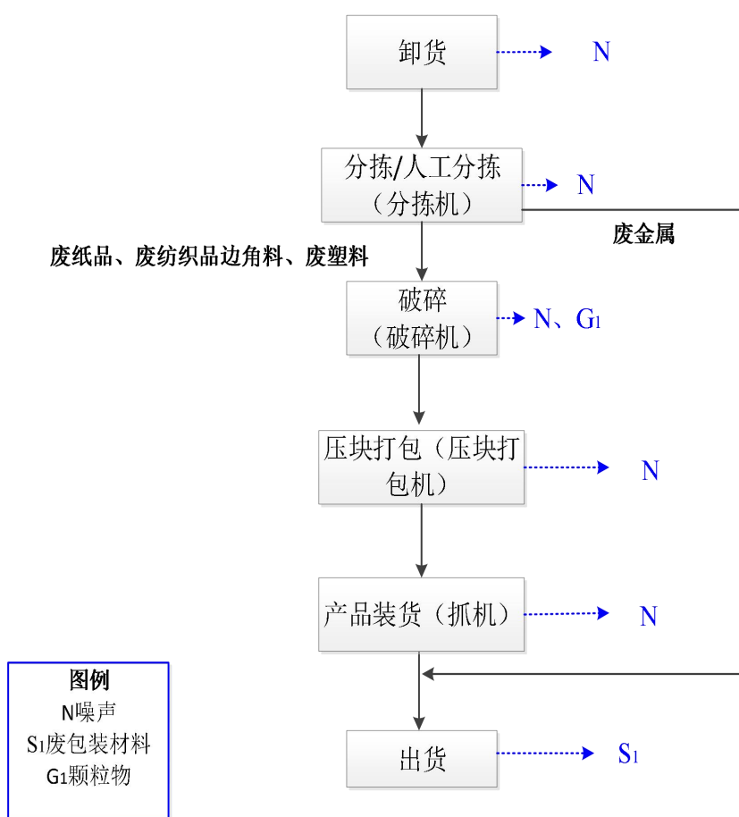
图 4 一般工业固体废物处理流程图
