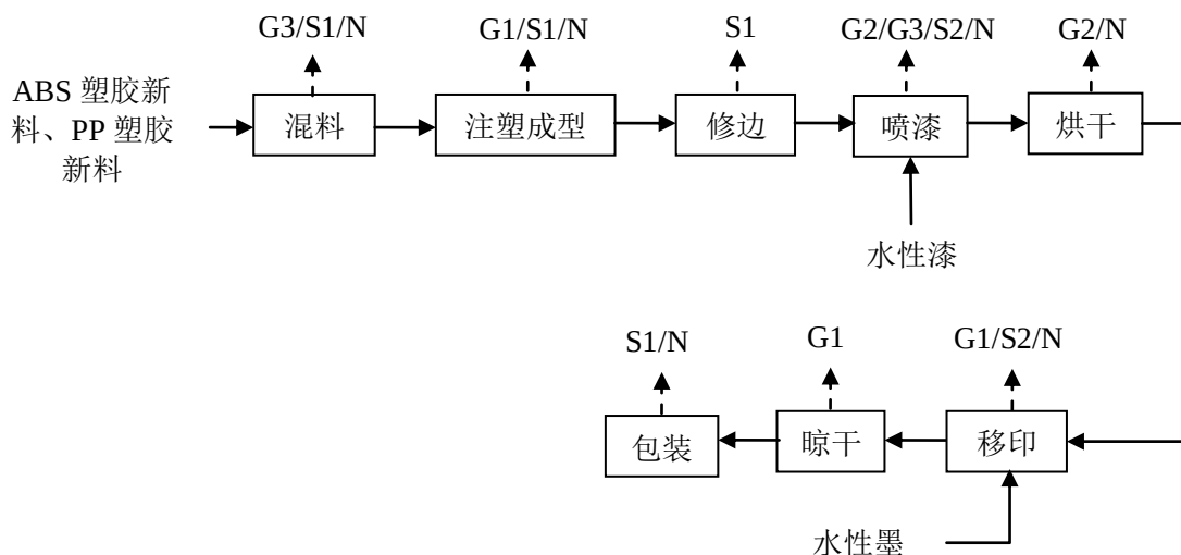
图 2 塑料制品、电动自行车外壳生产工艺及产污环节流程示意图
