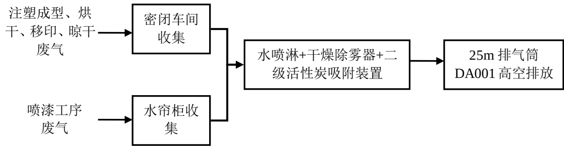
图 4 项目废气处理工艺流程图
