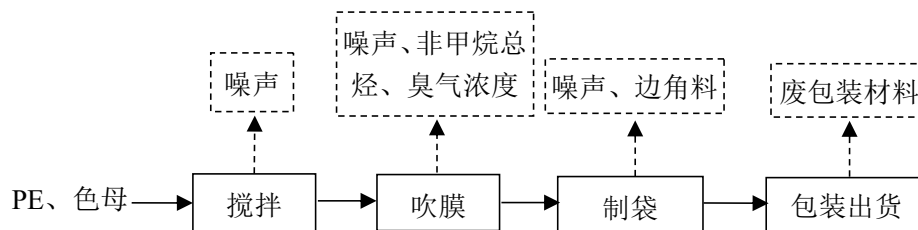
图 2-2 产品生产工艺流程图
