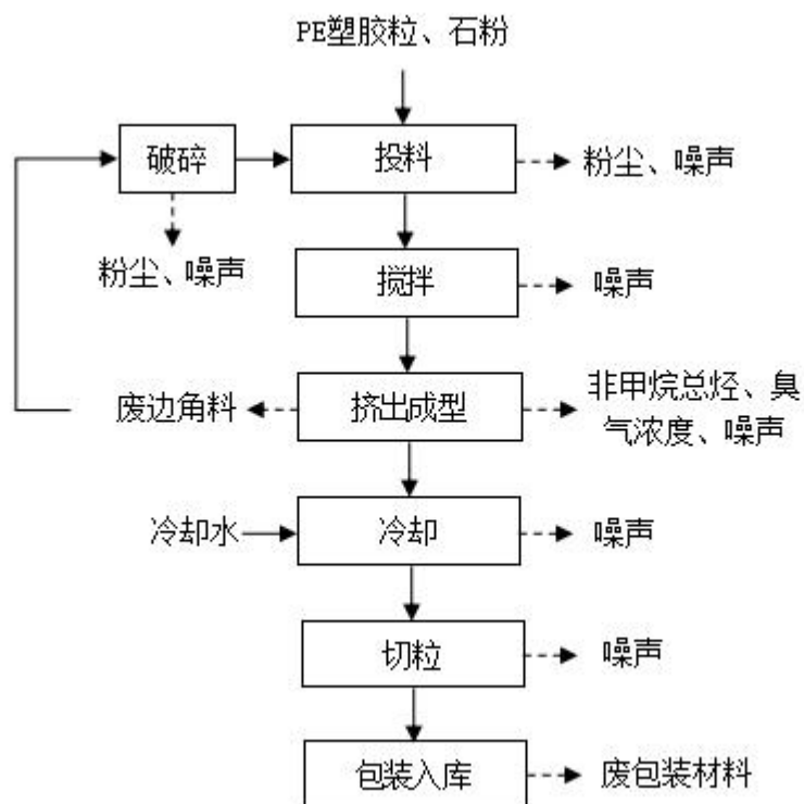
图 2-2 项目生产工艺流程图
