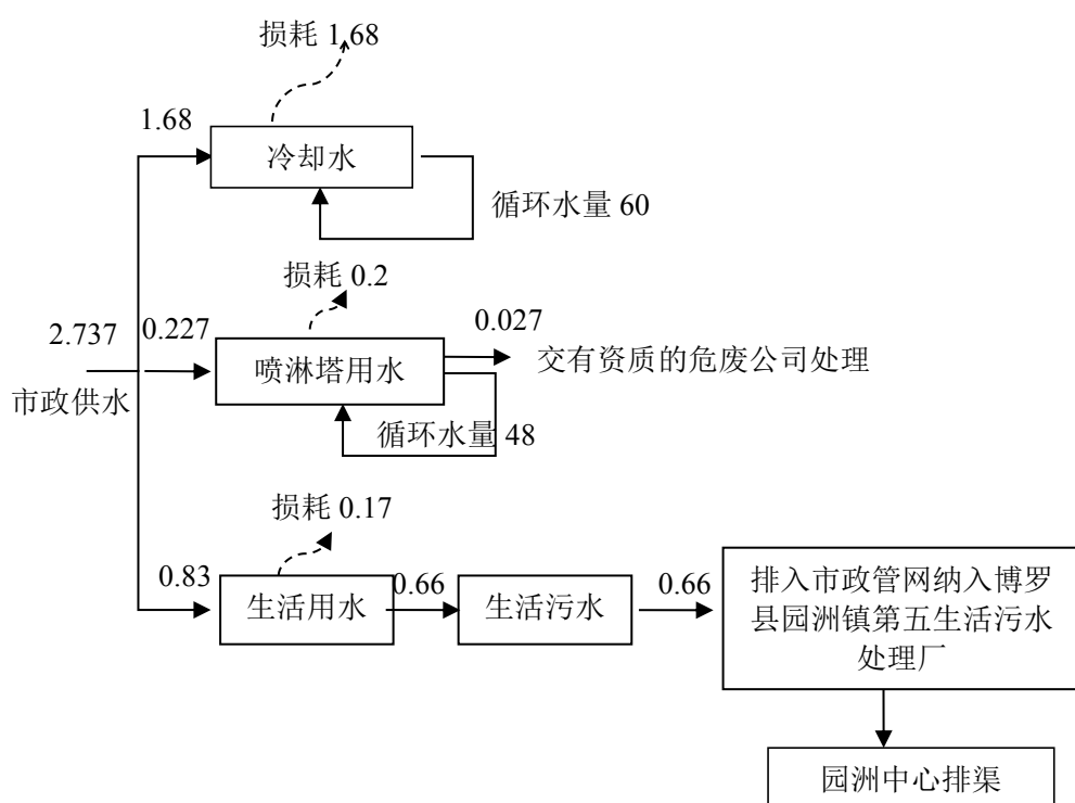
图 2-1 项目水平衡图（ \text{m}^3/\text{d} ）
