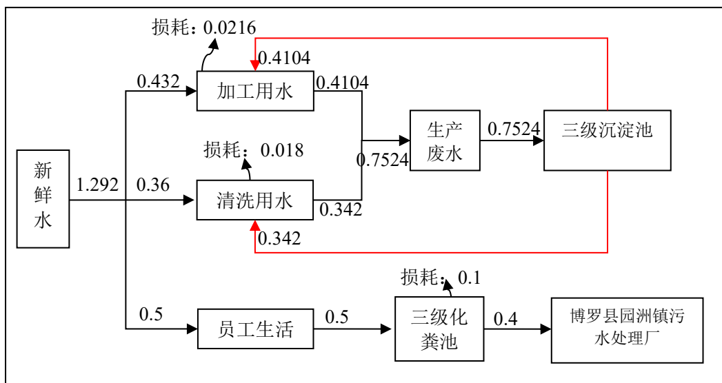
图1 本项目水平衡图 t/d
