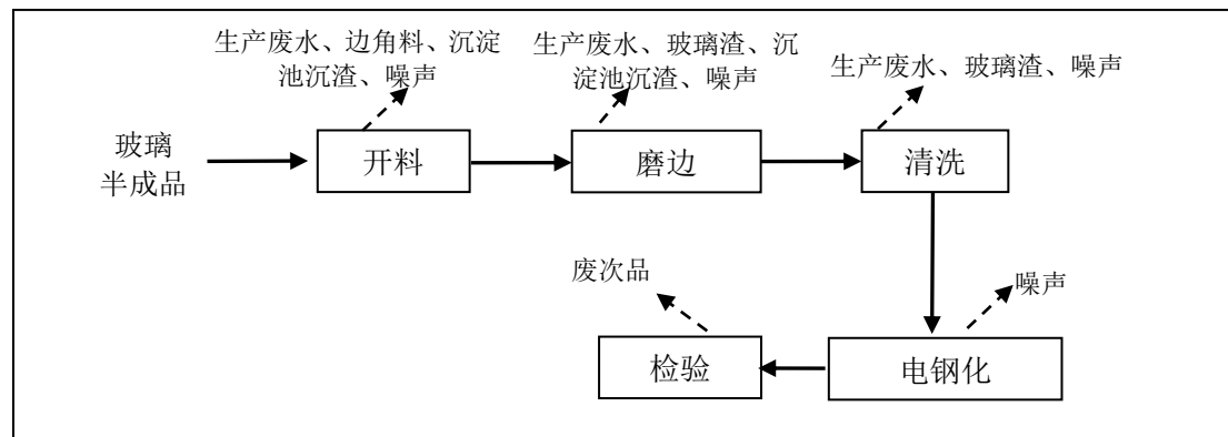
图3 项目主要工艺流程及产污环节分析示意图
