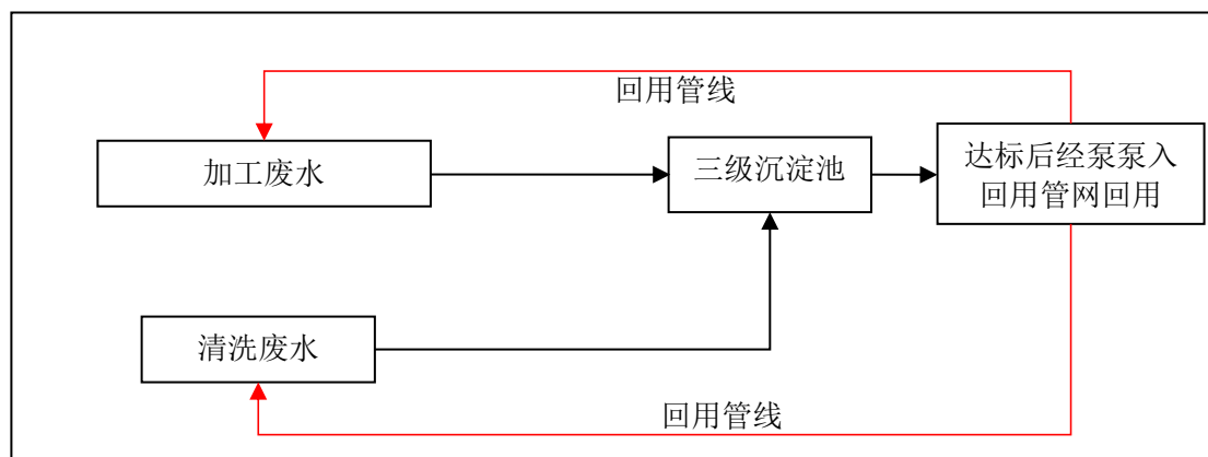
图 6 生产废水处理工艺流程图
