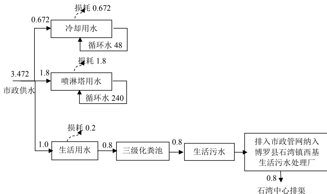
图 2-1 项目水平衡图 单位: \text{m}^3/\text{d}
