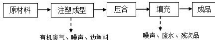
图 4 原有项目苹果手机外壳工艺流程图
