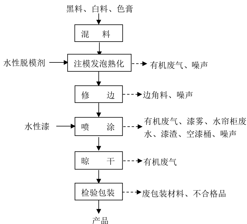
图 2 本项目生产工艺流程图
