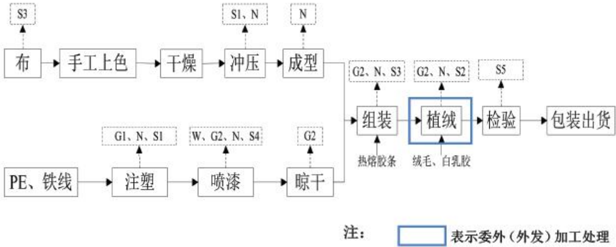
图 2-8 项目仿真花（塑料叶子）生产工艺流程图
