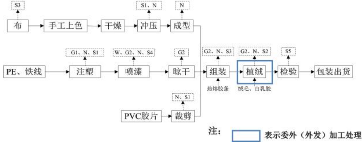
图 2-8 项目仿真花（PVC 片叶子）生产工艺流程图
