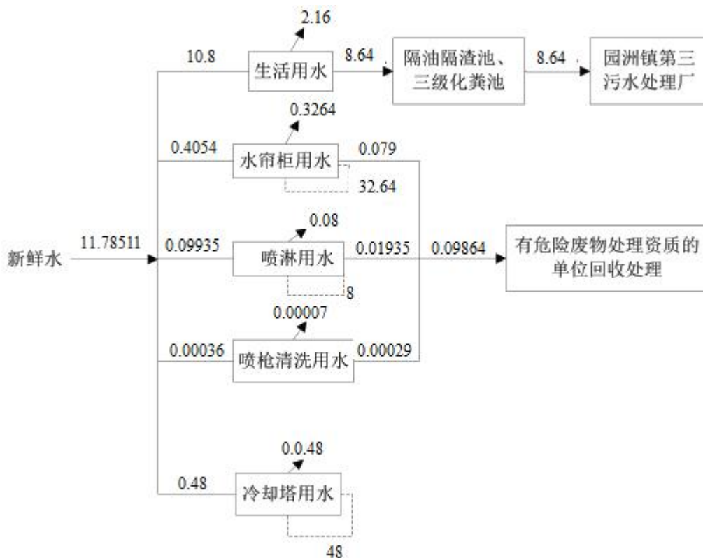
图 2-3 扩建后项目水平衡图 (t/d)
