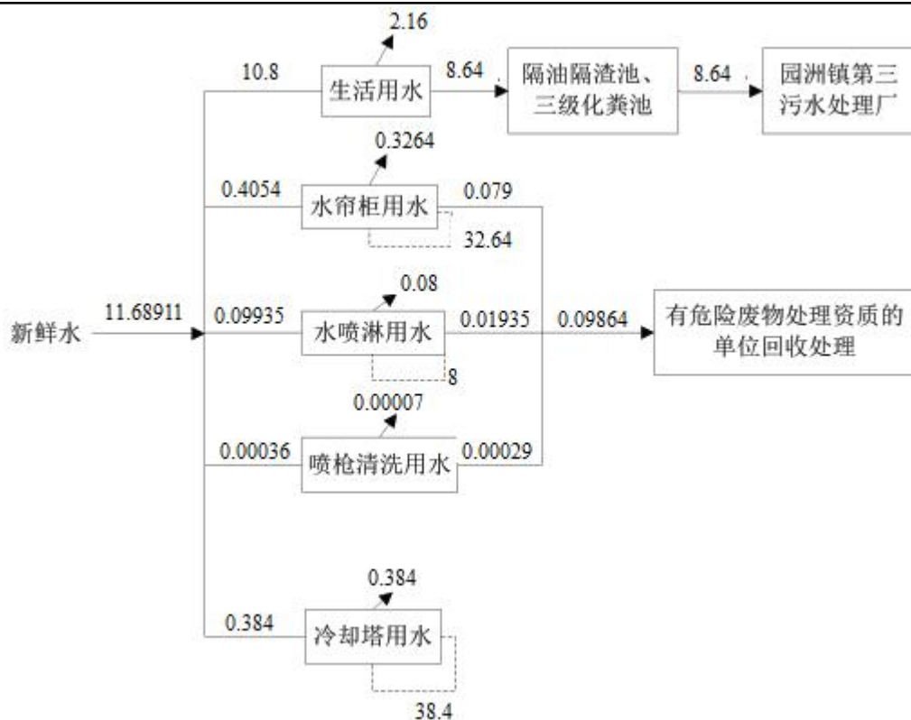
图 2-1 现有项目水平衡图 (t/d)
