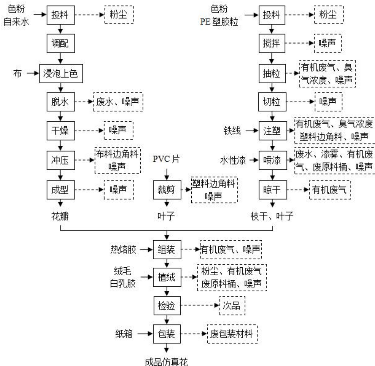
图 2-4 项目仿真花生产工艺流程图
