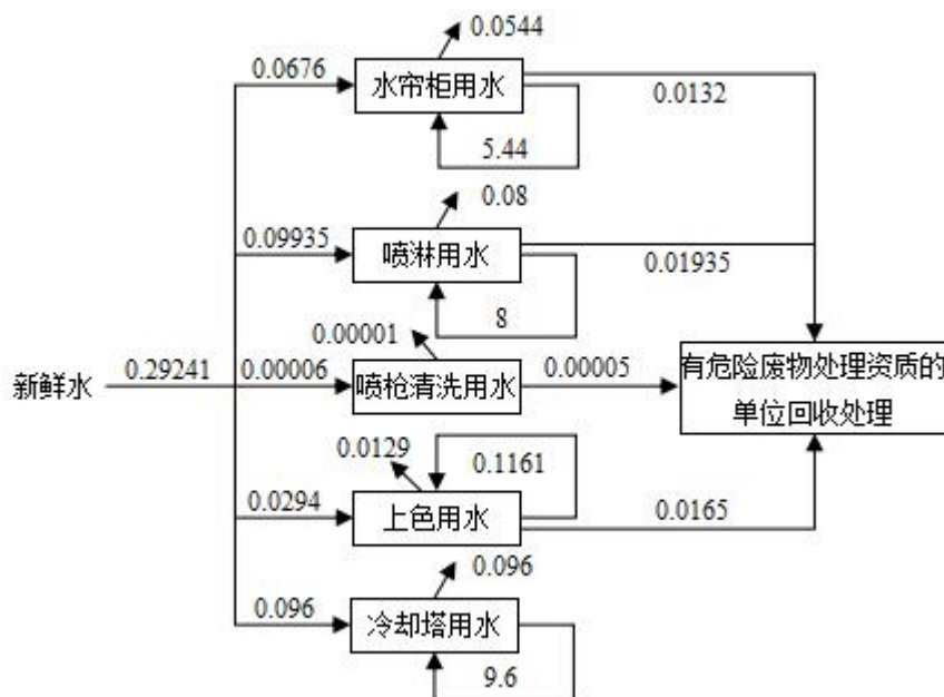
图 2-2 扩建项目水平衡图 (t/d)
