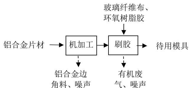
图 2-4 模具生产工艺流程图
