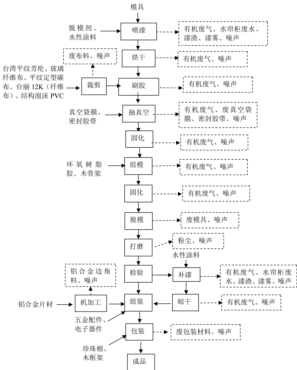
图 2-2 无人机机壳生产工艺流程图
