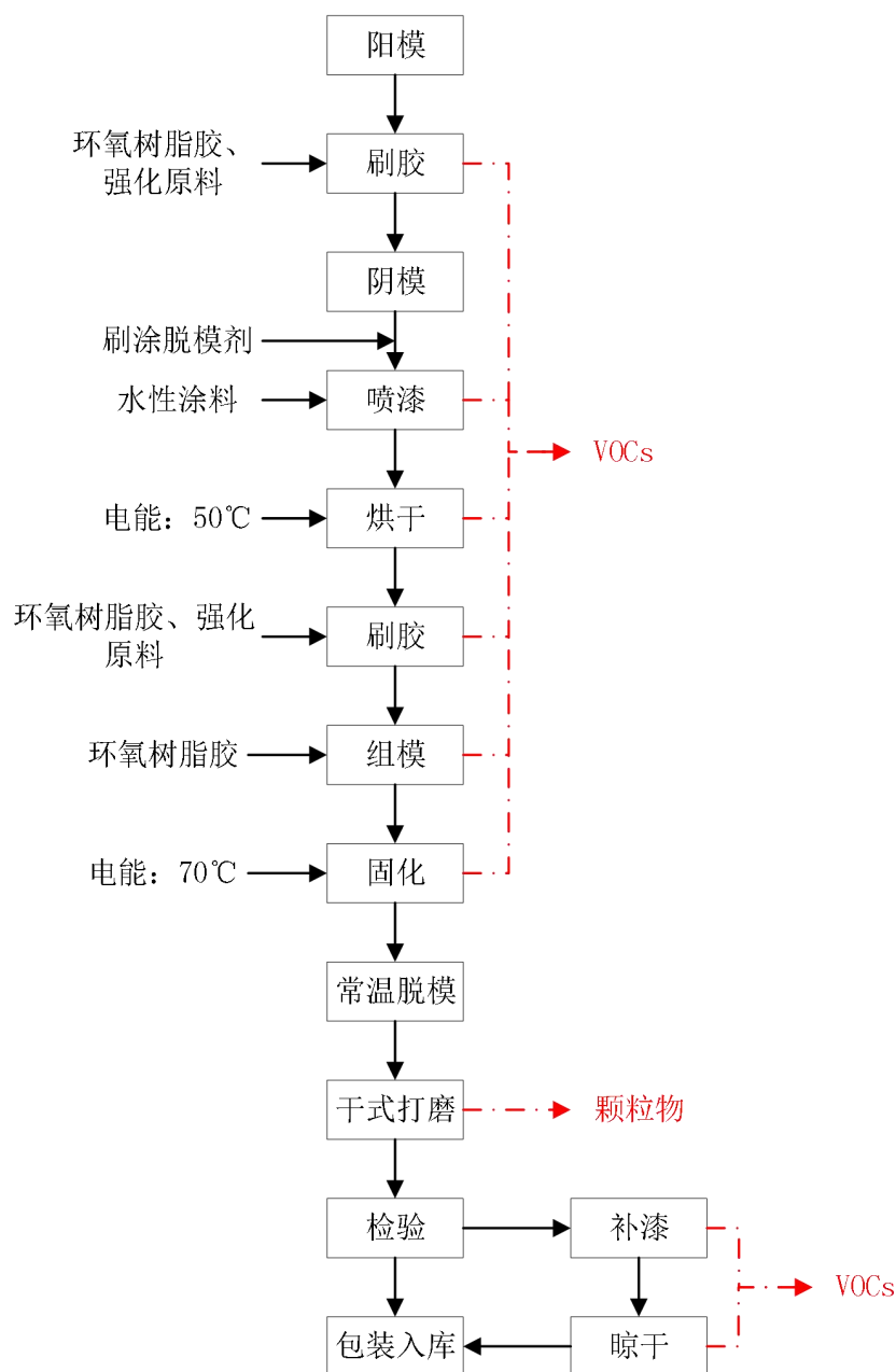
图 2-5 项目原有产品生产工艺流程图
