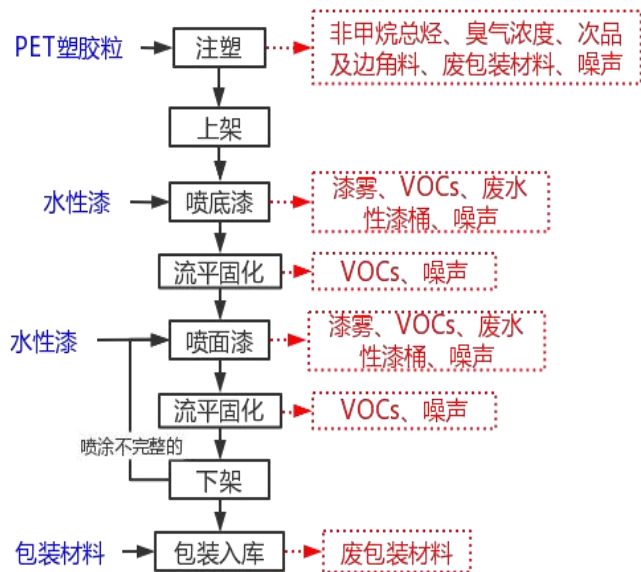
图 2-3 项目塑胶件生产工艺流程图
