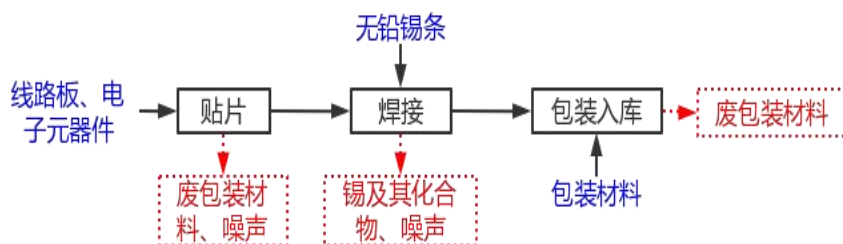
图 2-4 项目线路板生产工艺流程图
