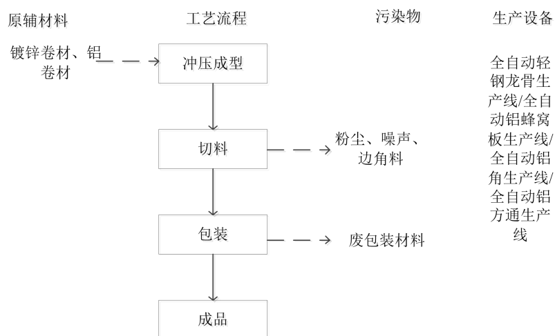
图 3 铝方通和镀锌龙骨生产工艺
