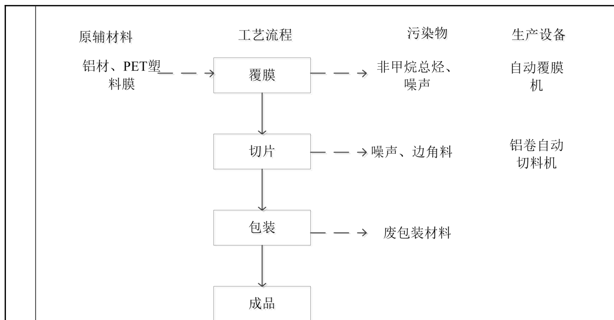
图 4 覆膜铝板生产工艺
