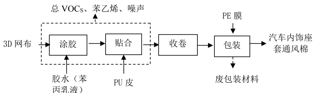
图 2-3 项目汽车内饰座套通风棉生产工艺流程图
