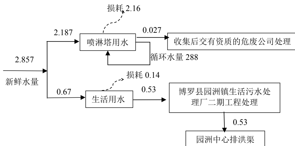
图 2-2 项目水平衡图 ( \text{m}^3/\text{d} )
