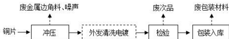
图 2-3 项目集成电极生产工艺流程及产污环节图
