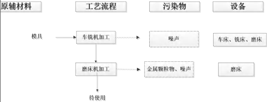
图 2-5 项目模具维修生产工艺流程图
