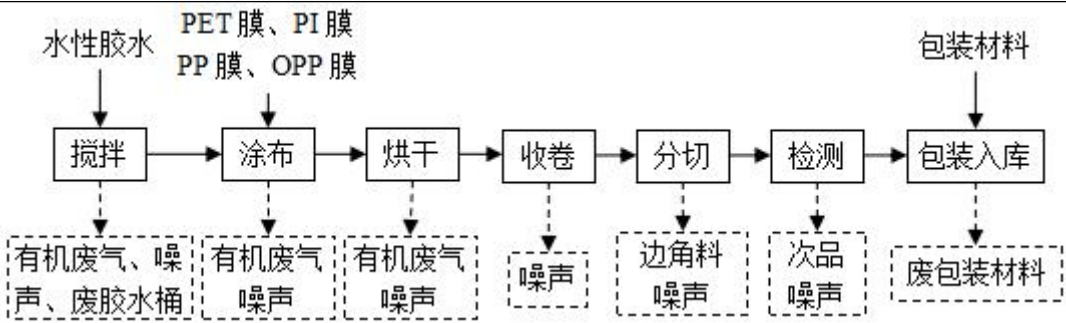
图 2-2 项目工艺流程及产污环节图
