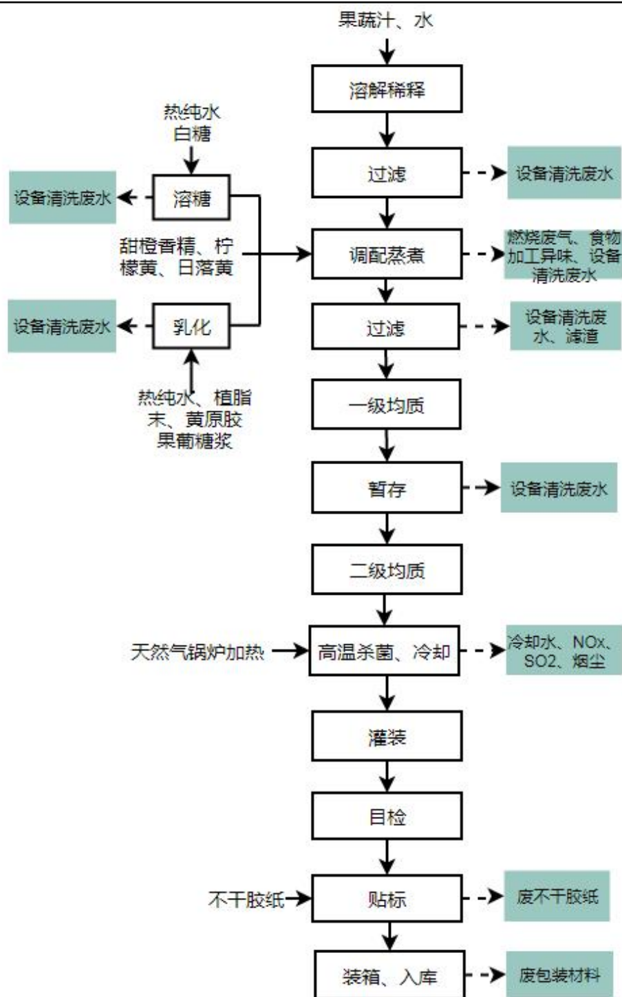
图 2-6 改扩建项目果蔬饮料生产工艺流程图
