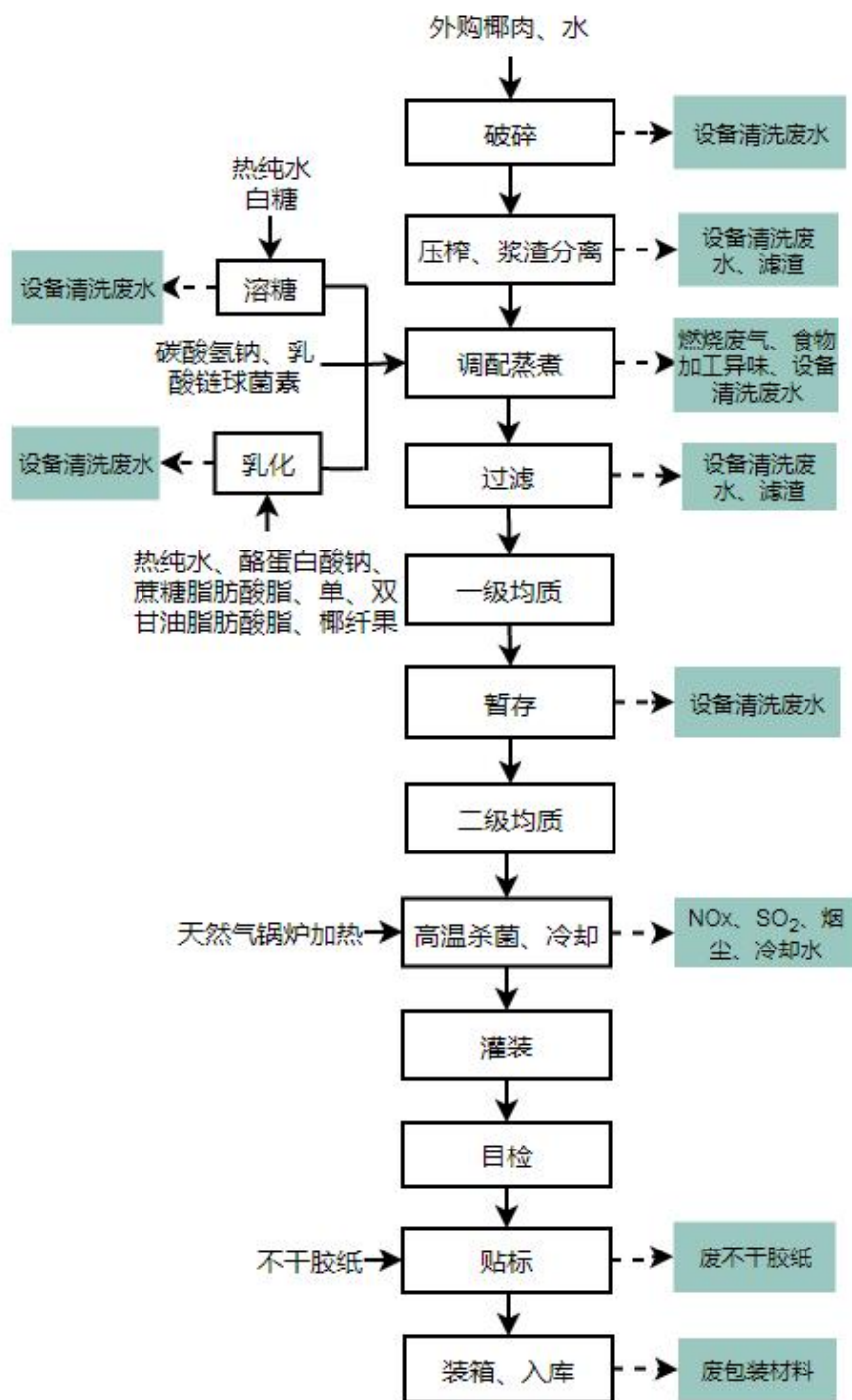
图 2-4 改扩建项目椰汁生产工艺流程图
