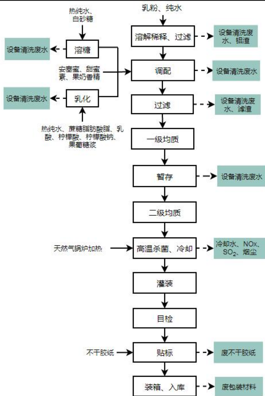
图 2-5 改扩建项目含乳饮料生产工艺流程图
