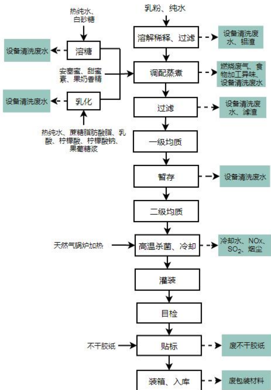
图 2-7 改扩建项目咖啡饮料生产工艺流程图
