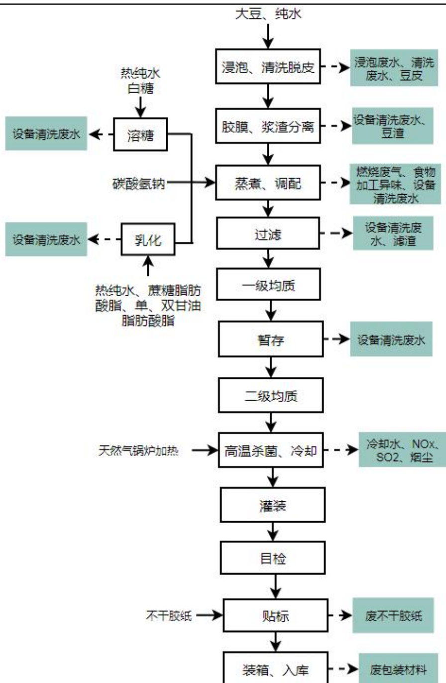
图 2-3 改扩建项目豆奶生产工艺流程图
