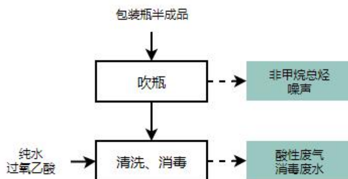
图 2-8 改扩建项目吹瓶工序生产工艺流程图
