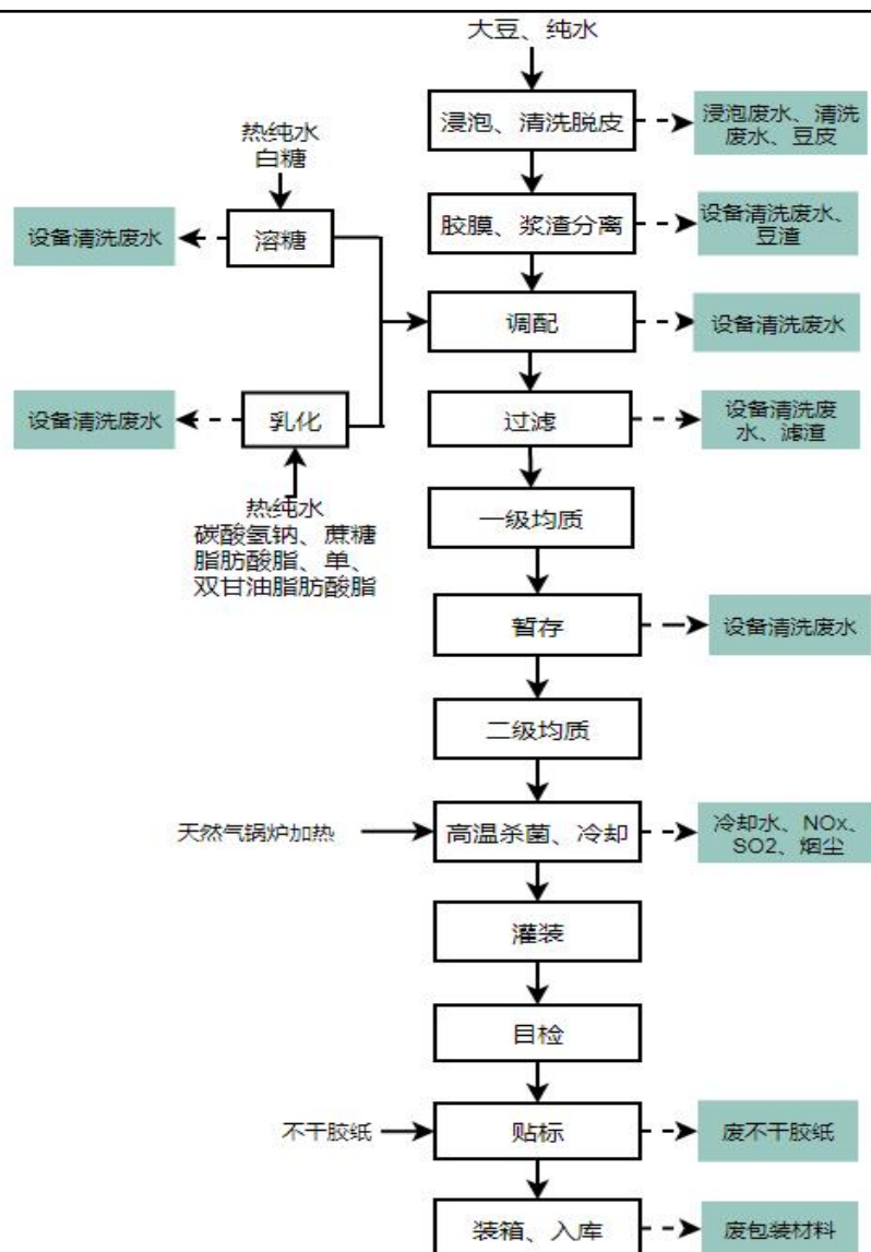
图 2-9 现有项目豆奶工艺流程图
