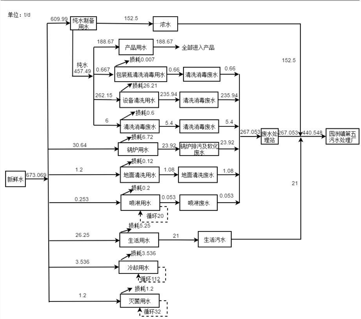
图2-2 改扩建后全厂总水平衡图
