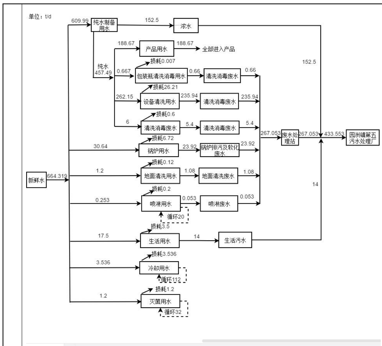
图2-1 改扩建项目水平衡图
