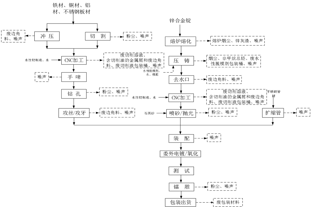
图 2 五金产品及配件生产工艺流程图及产污环节
