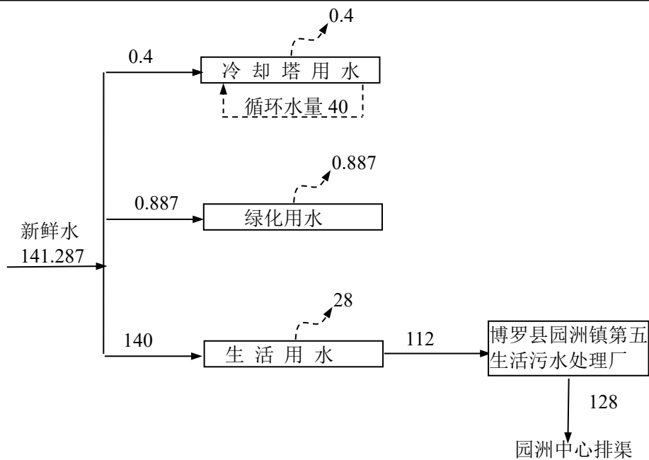
图 1 项目日水平衡图 (t/d)
