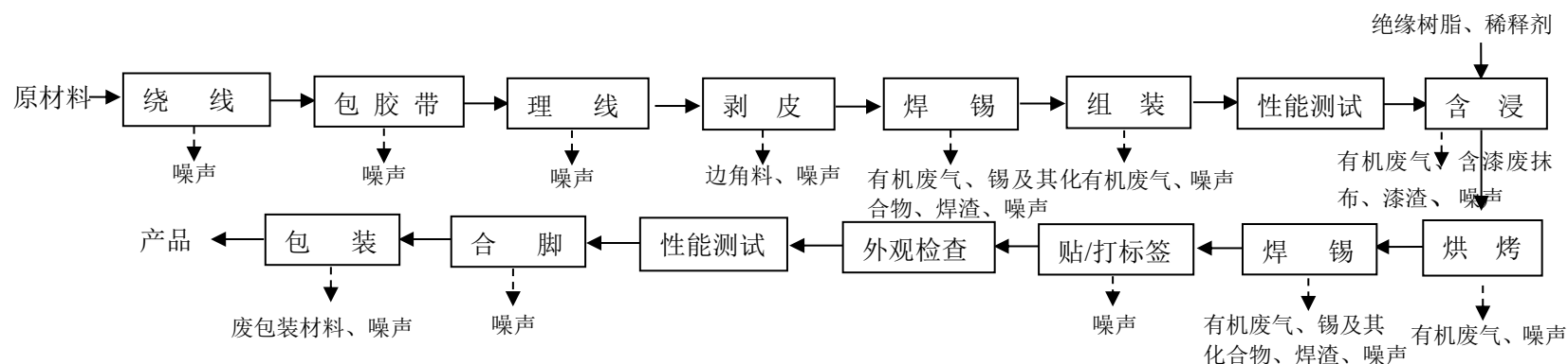
图3 项目变压器生产工艺流程图
