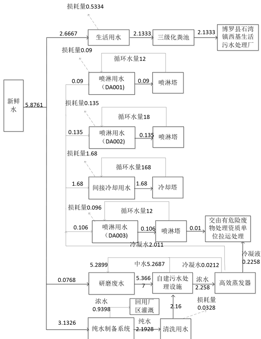
图1 改扩建后全厂项目水平衡图 (t/d)
