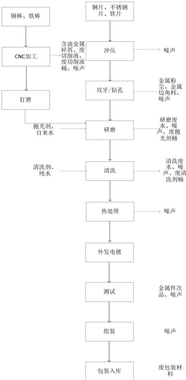
图 2 五金配件生产工艺流程图
