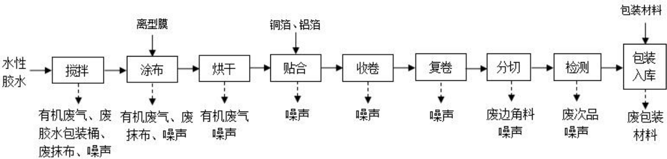
图 2-3 项目铜箔胶带、铝箔胶带生产工艺流程图
