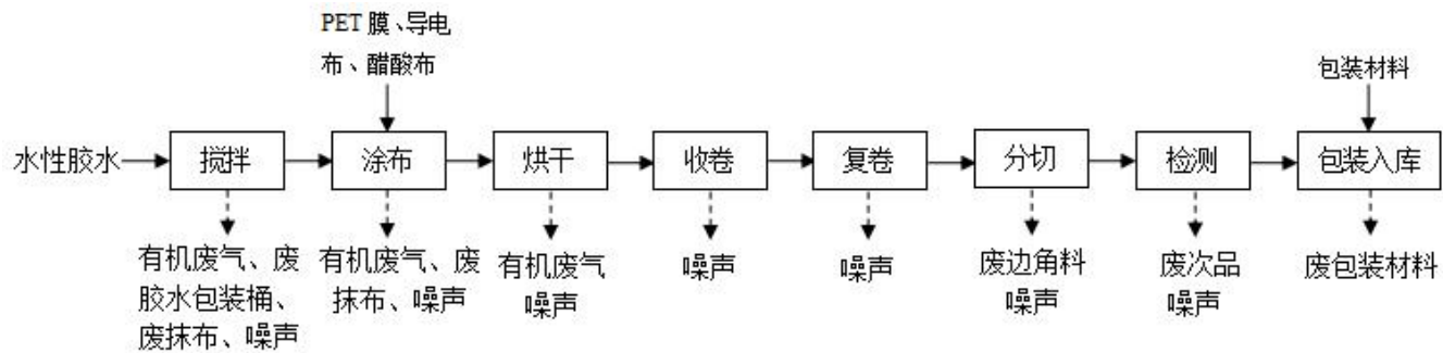
图 2-2 项目 PET 胶带、导电布胶带、醋酸布胶带生产工艺流程图
