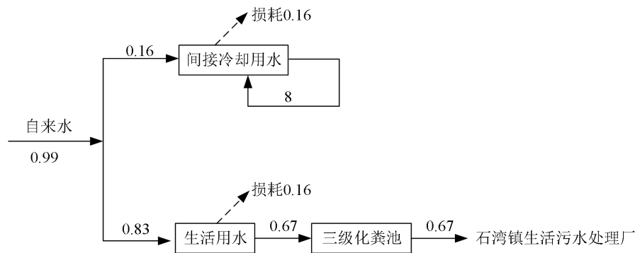
图 1 项目水量平衡图（单位：t/d）
