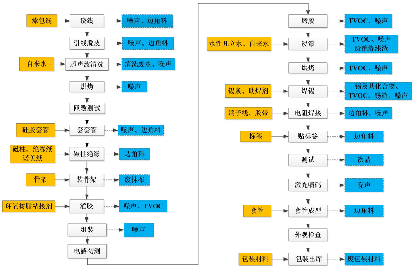
图 2-4 项目变压器生产工艺流程及产污环节示意图
