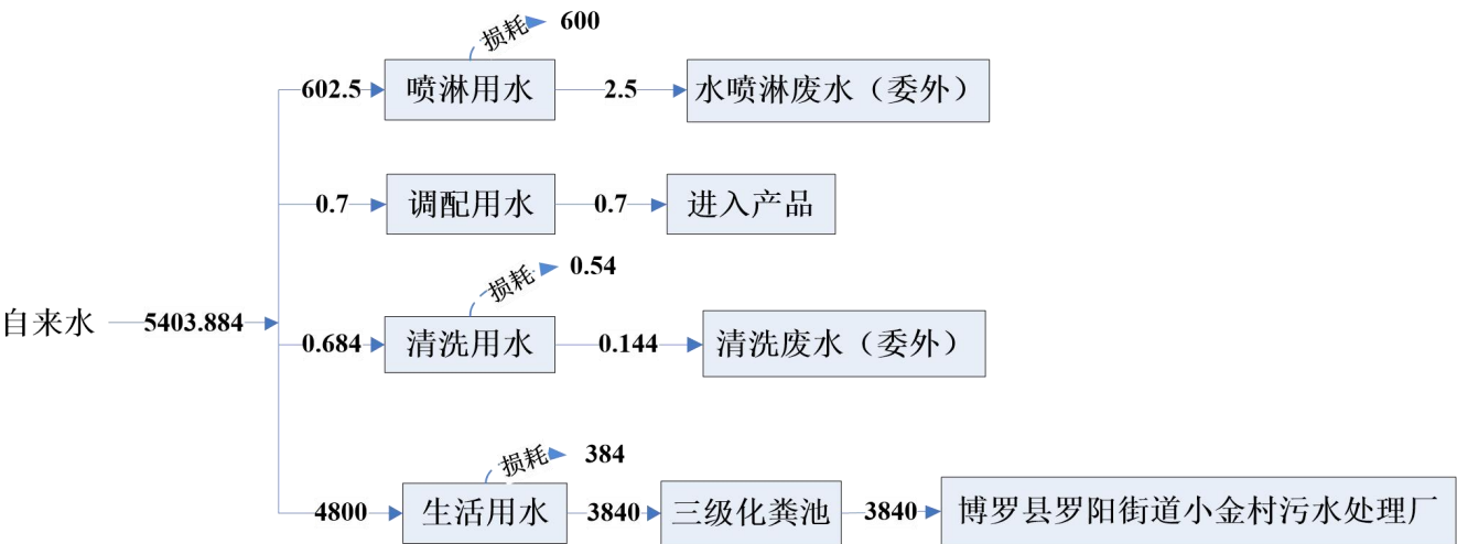
图 2-2 项目水平衡示意图 单位：m³/a
