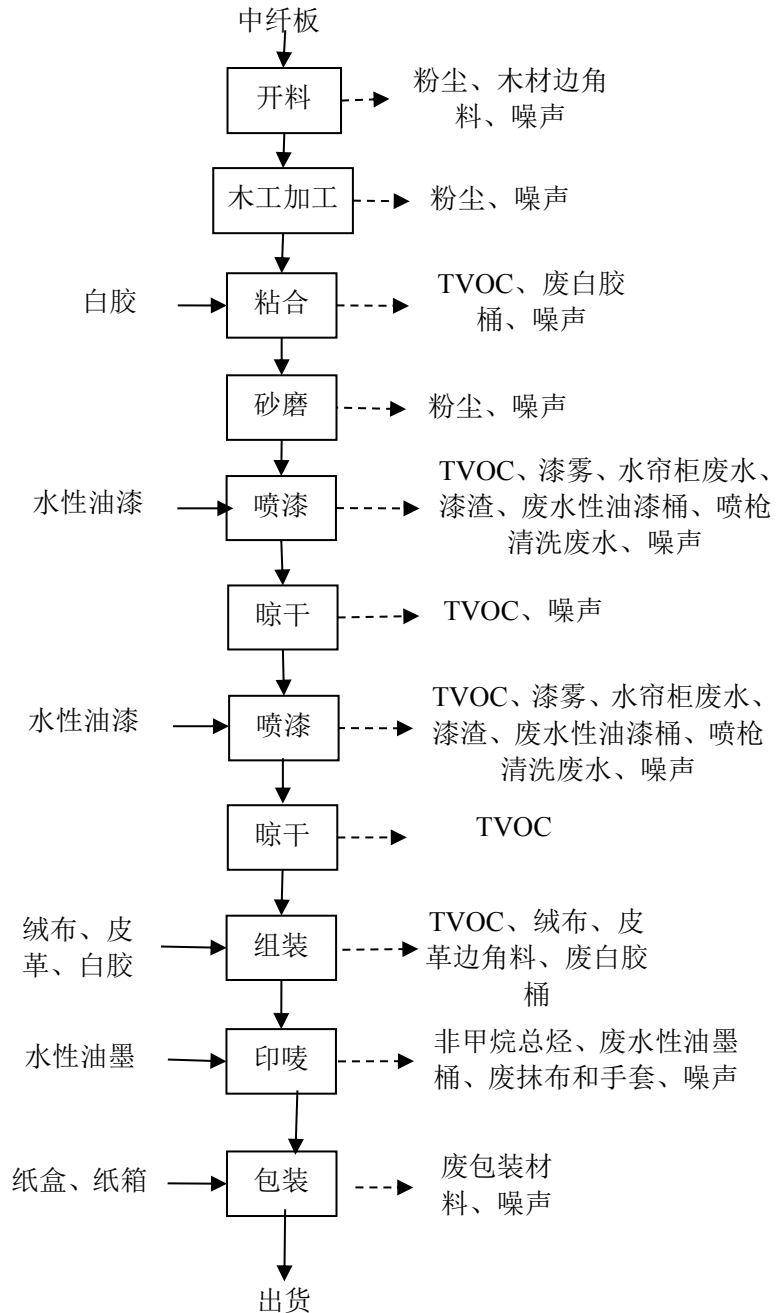
2-2 项目木盒生产工艺流程图
