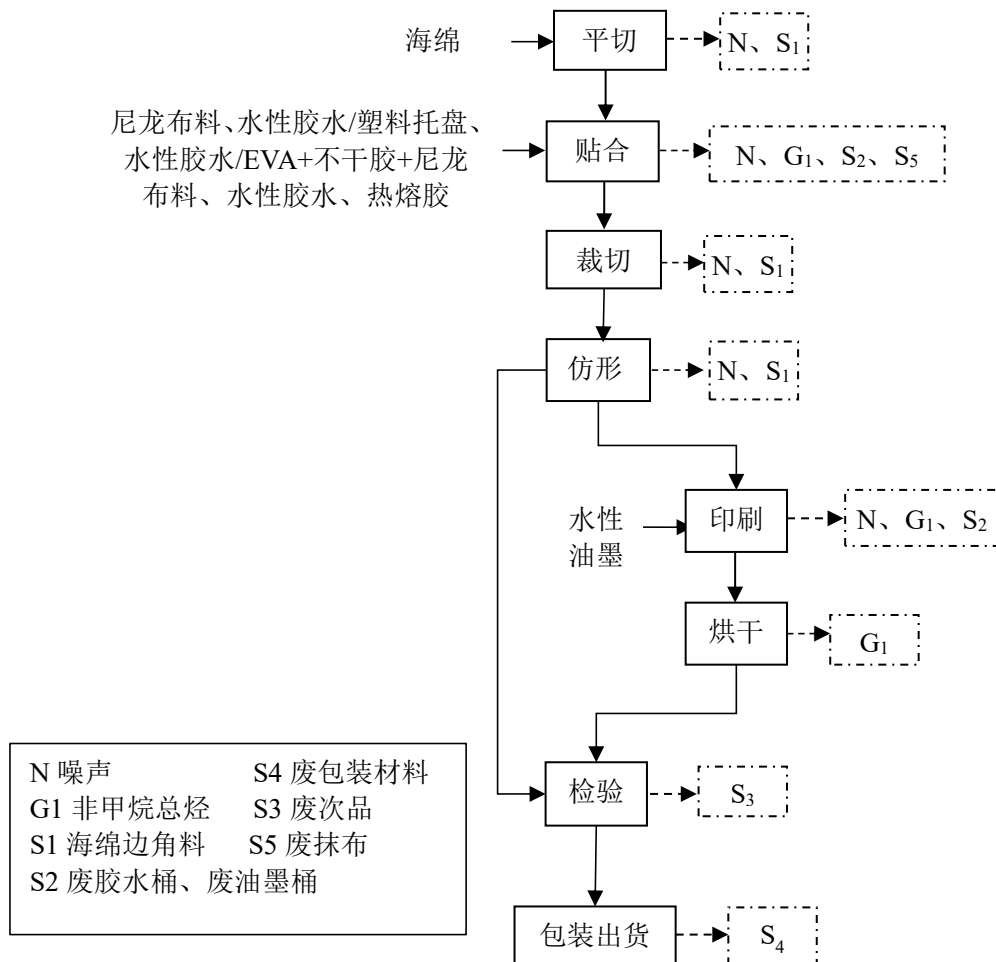
图2 汽车抛光用海绵产品工艺流程及产污环节分析示意图
