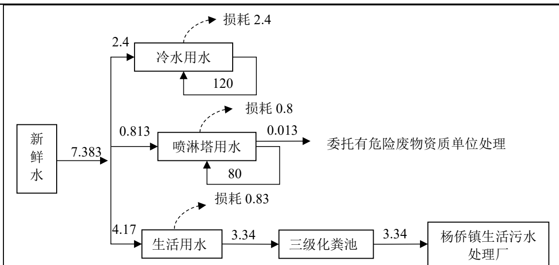
图1 项目水平衡示意图 单位: \text{m}^3/\text{d}
