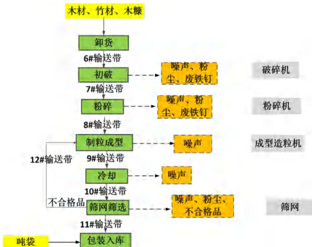
图 2-3 项目生物质成型颗粒生产工艺流程图
