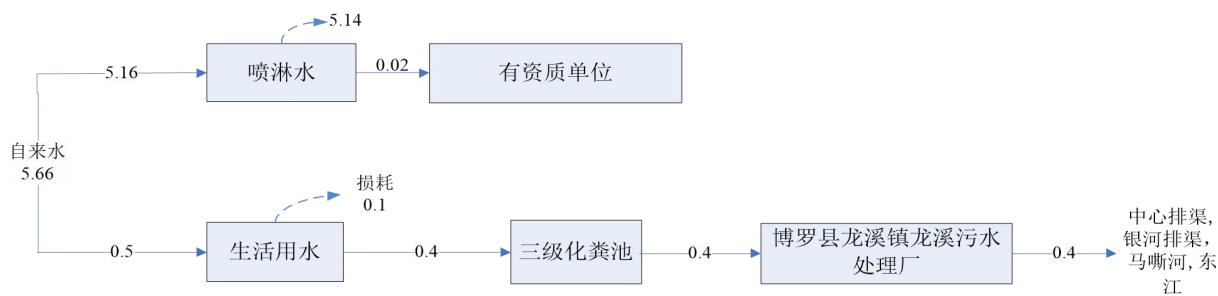
图 2-2 项目水平衡图 (单位 t/d)
