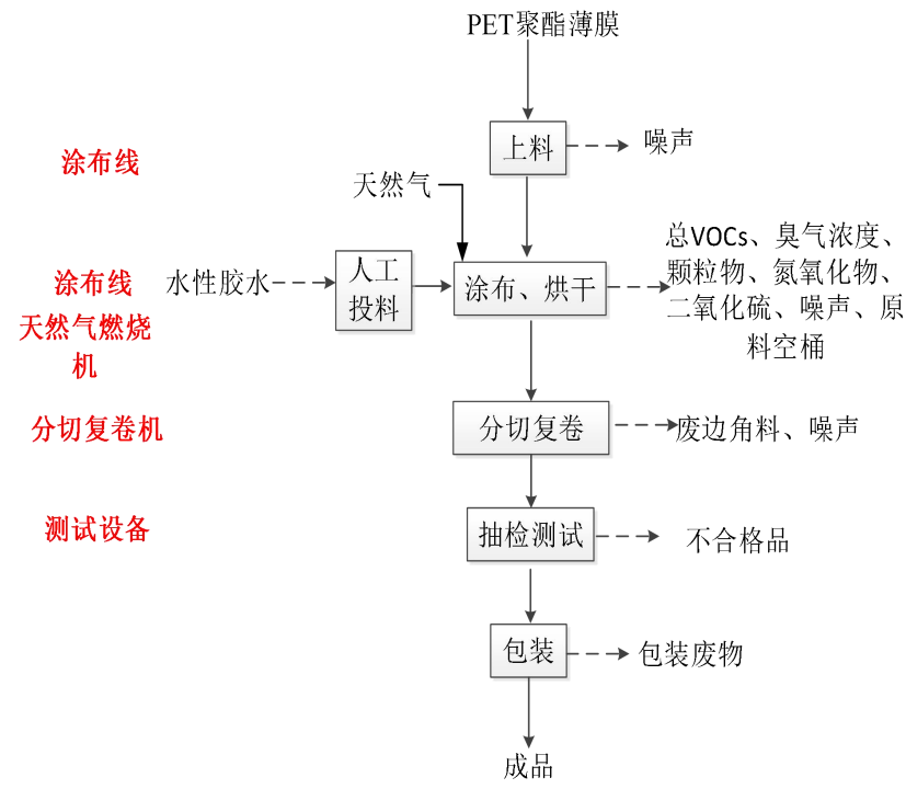
图 2-4 项目离型膜生产工艺流程
