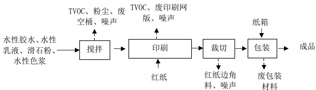
图 2-3 对联生产工艺流程图
