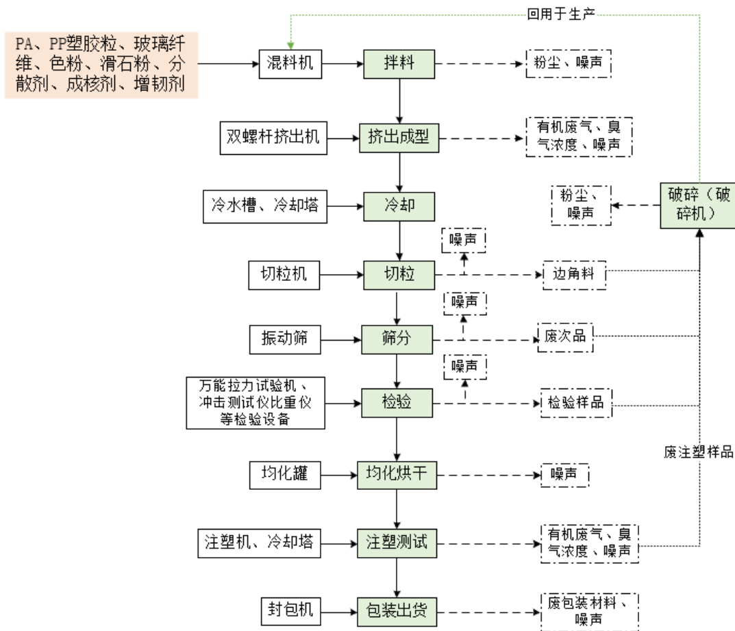
图2 项目工艺流程及产污环节分析示意图
