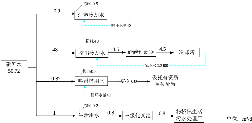
图1 项目水平衡示意图
