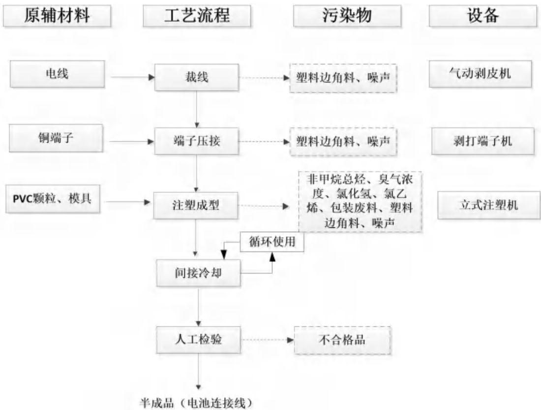
图 2-4 项目半成品（电池连接线）生产工艺流程图
