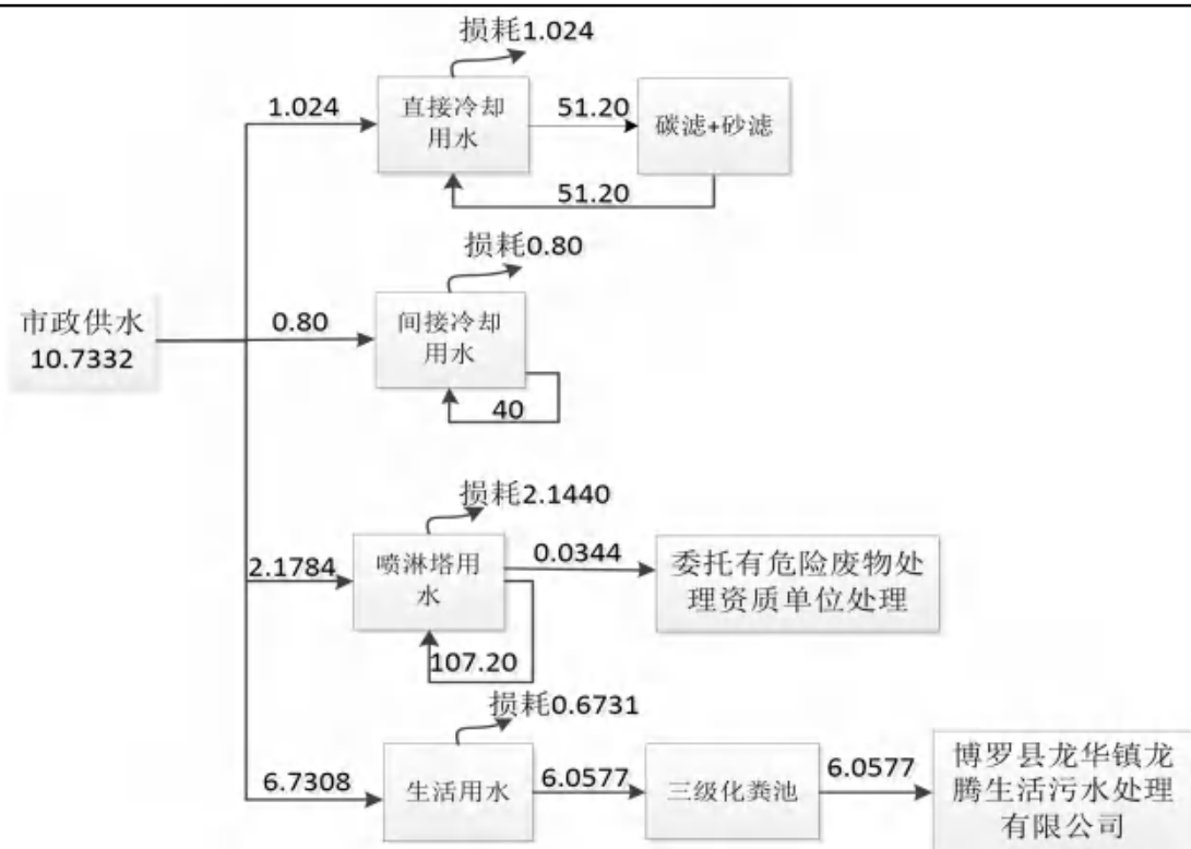
图 2-2 扩建后项目水平衡图 单位：t/d
