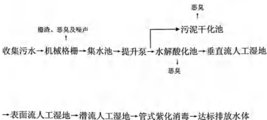
图 4-1 博罗县龙华镇龙腾生活污水处理有限公司工艺流程图
