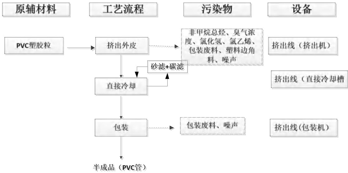
图 2-3 项目半成品（PVC 管）生产工艺流程图
