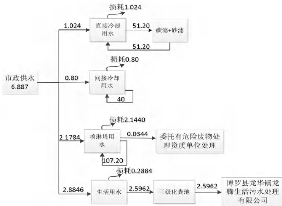
图 2-1 扩建项目水平衡图 单位：t/d
