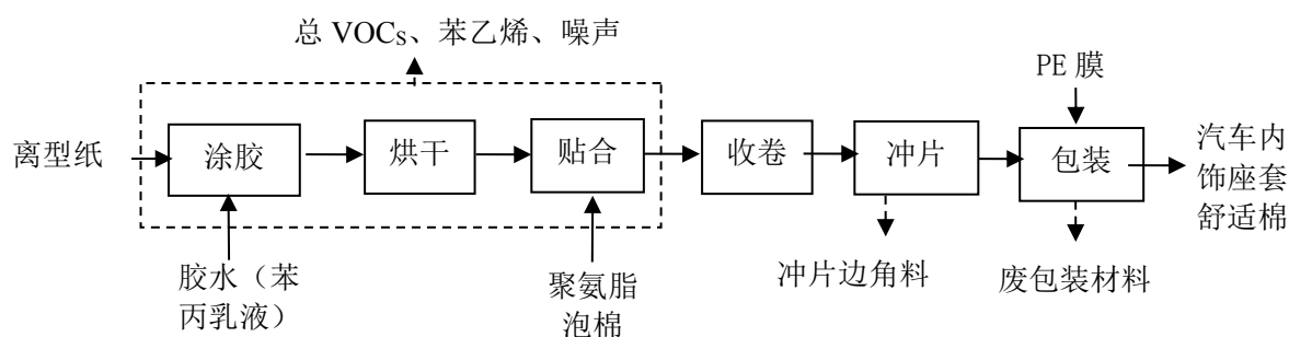
图 2-4 项目汽车内饰座套舒适棉生产工艺流程图
