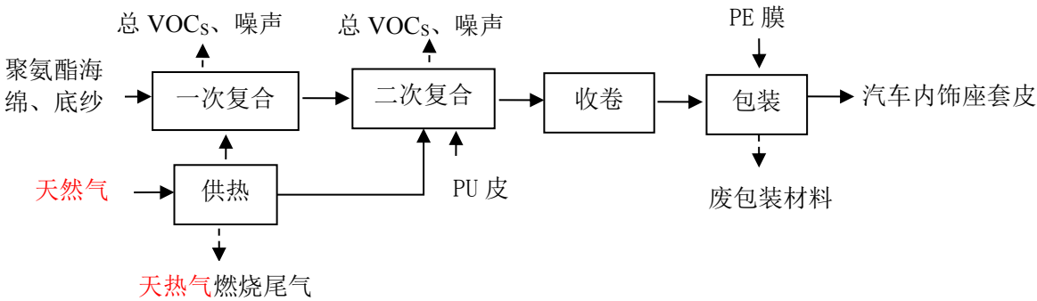
图 2-2 项目汽车内饰座套皮生产工艺流程图
