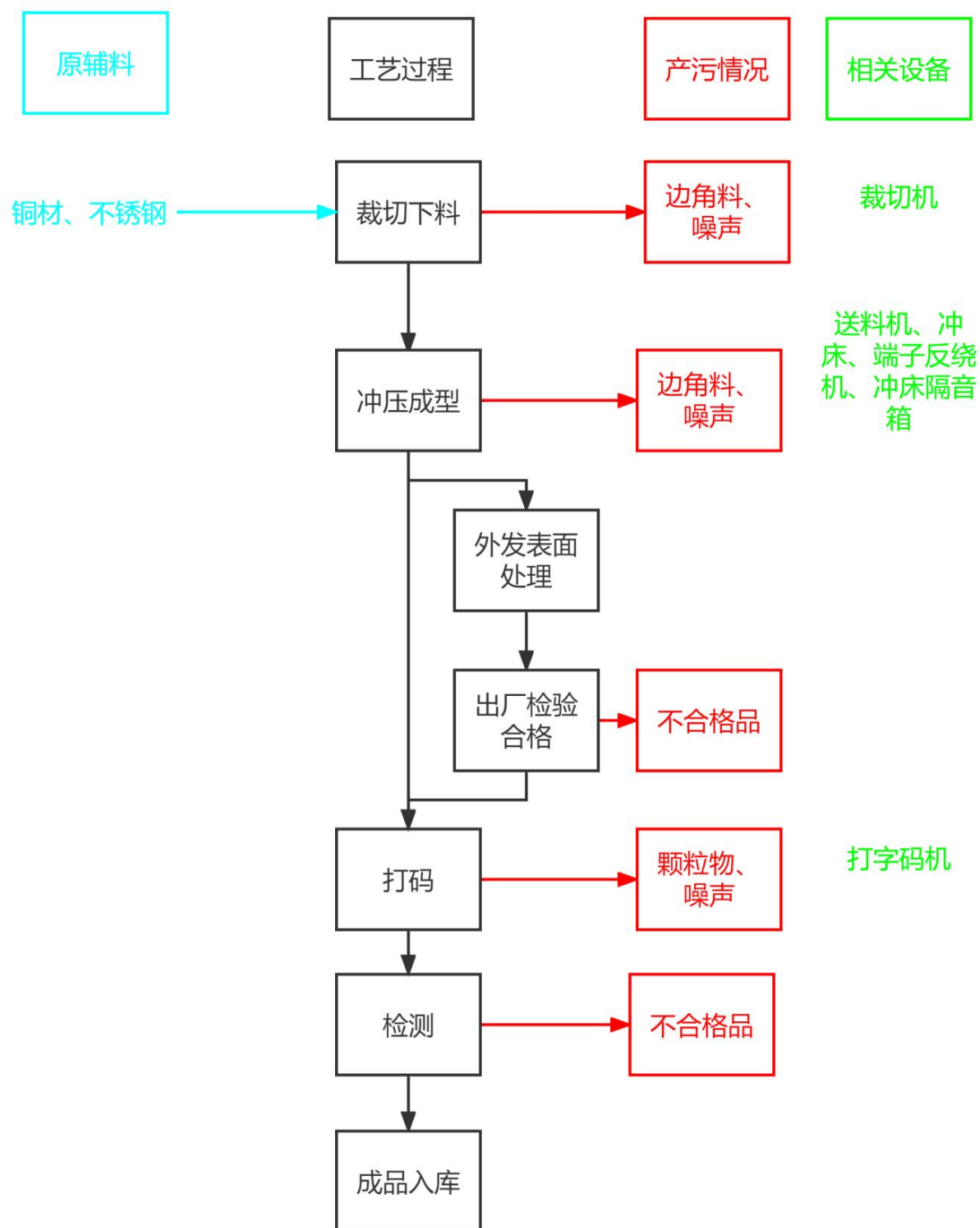
图 2-5 五金件工艺流程图
