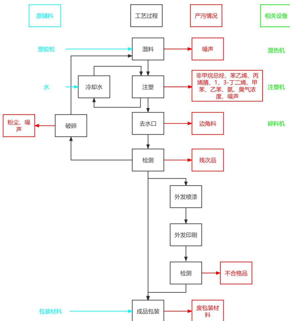
图 2-6 c 栋塑料外壳、塑料卷筒、塑料托盘工艺流程图
