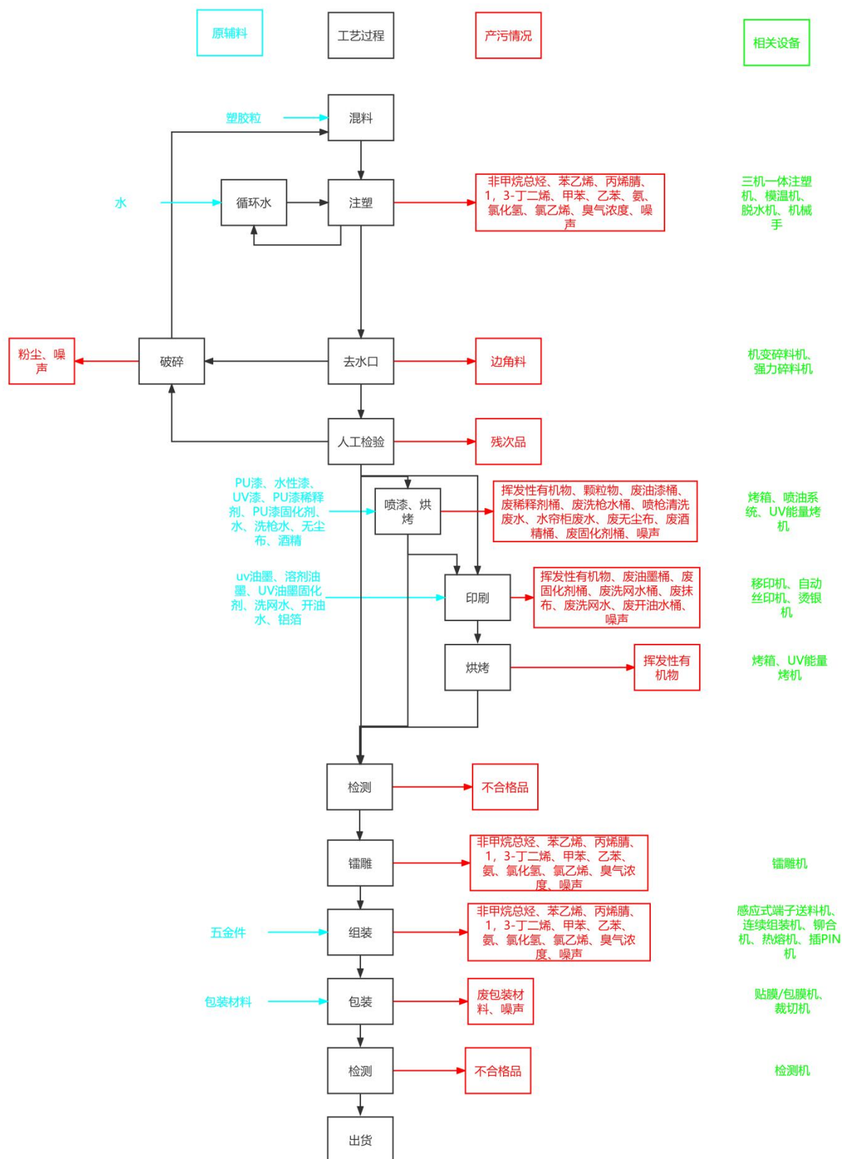
图2-3 塑料外壳、产成品的工艺流程图
