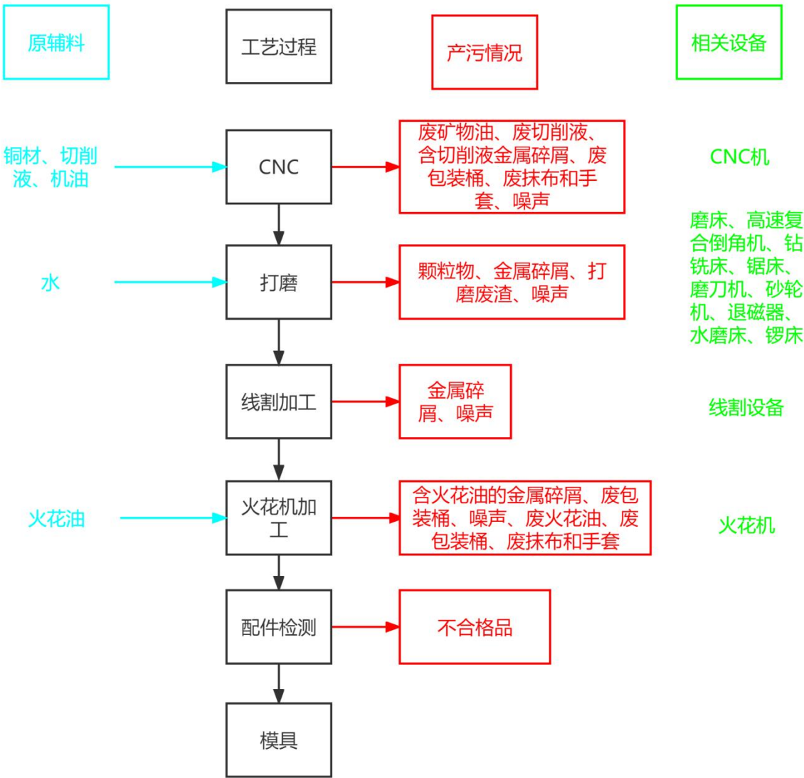
图2-4 模具的工艺流程图
