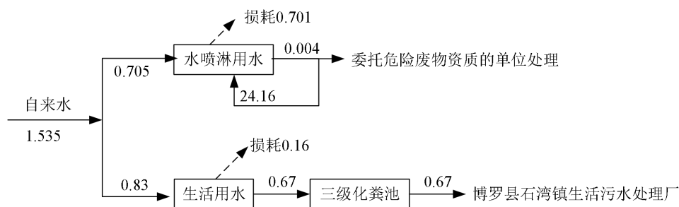
图 1 项目水量平衡图 (单位: t/d)
