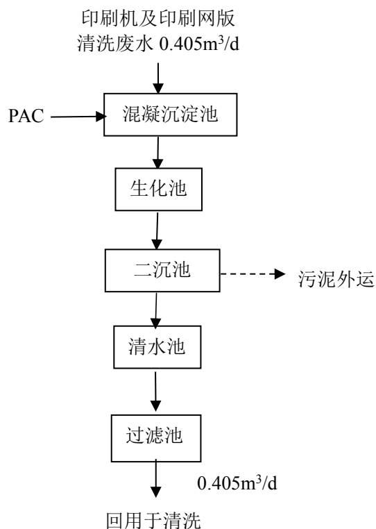
图 4-1 废水处理工艺流程图
