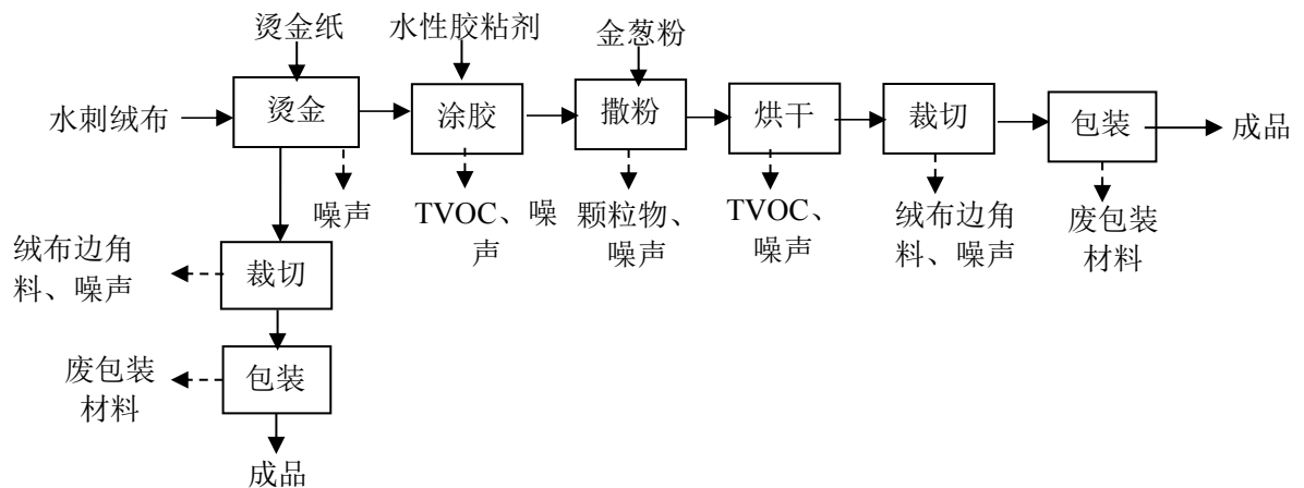
图 2-2 福字生产工艺流程图
