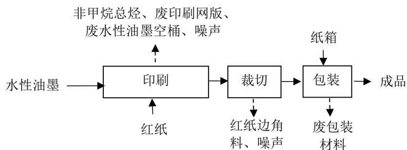
图 2-3 对联生产工艺流程图
