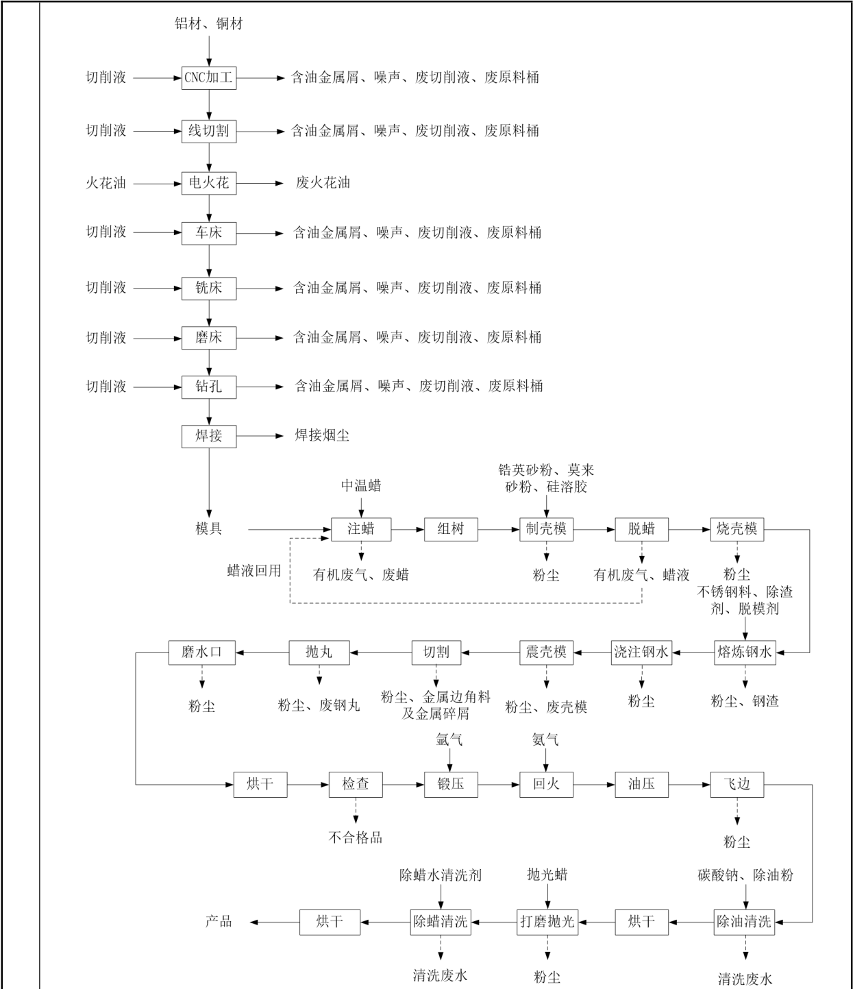
图5 现有项目生产工艺流程图
