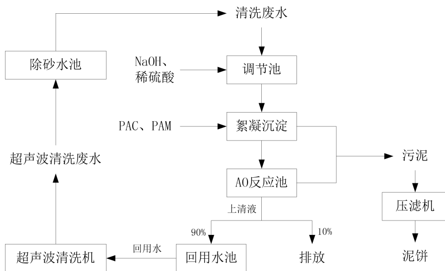
图7 自建污水处理设施处理工艺流程图
