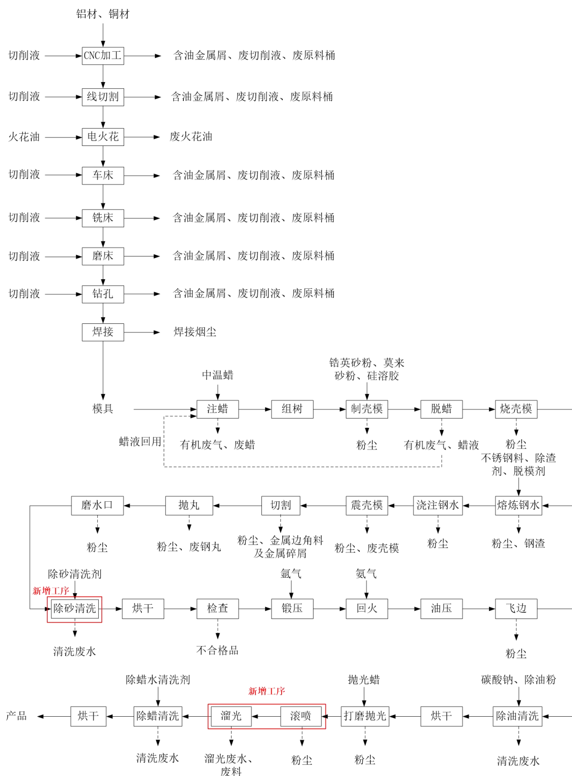
图 4 项目生产工艺流程图
