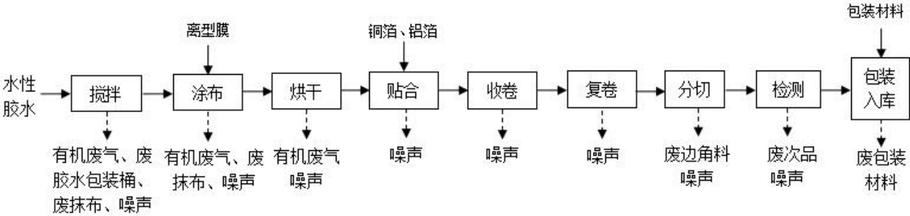
图 2-4 项目铜箔胶带、铝箔胶带生产工艺流程图
