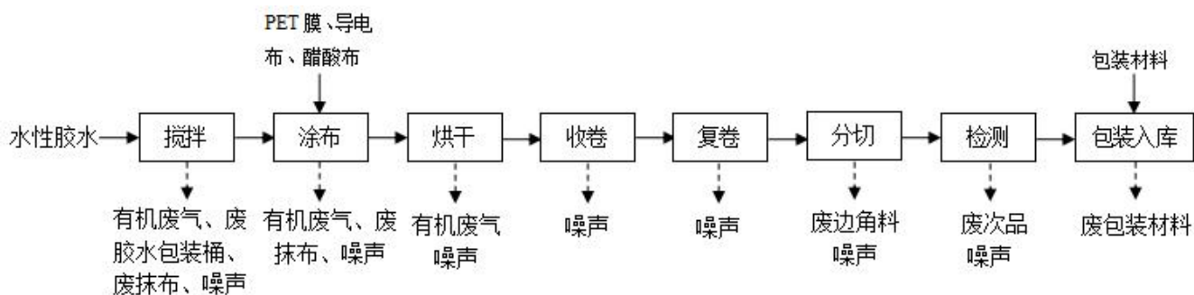
图 2-3 项目 PET 胶带、导电布胶带、醋酸布胶带生产工艺流程图
