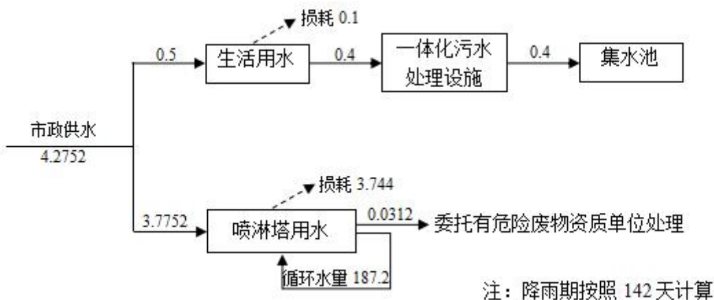
图 2-2 项目降雨期水平衡图 (t/d)
