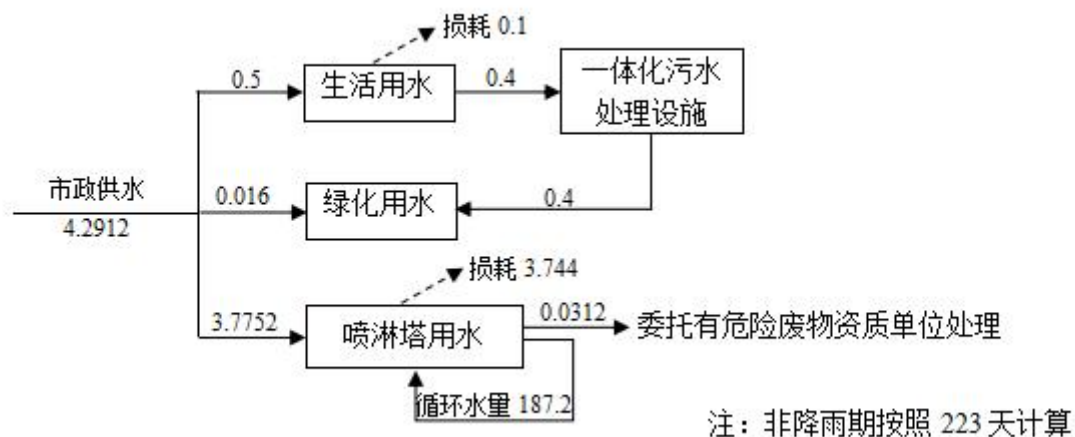
图 2-1 项目非降雨期水平衡图 (t/d)
