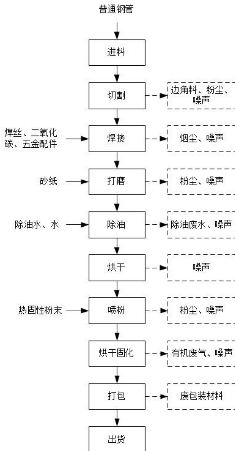
图2 工艺流程图
