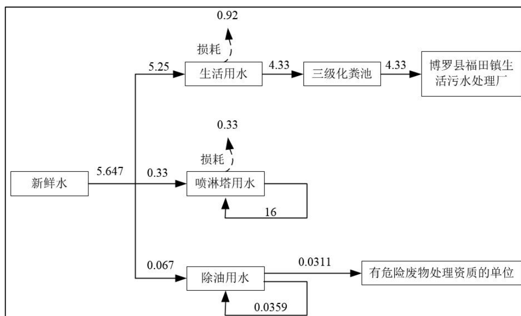
图 1 本项目水平衡图（t/d）
