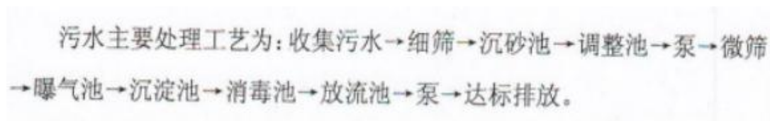
图4 污水处理工艺流程图
