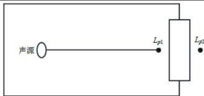
图 5 室内声源等效为室外声源图例
