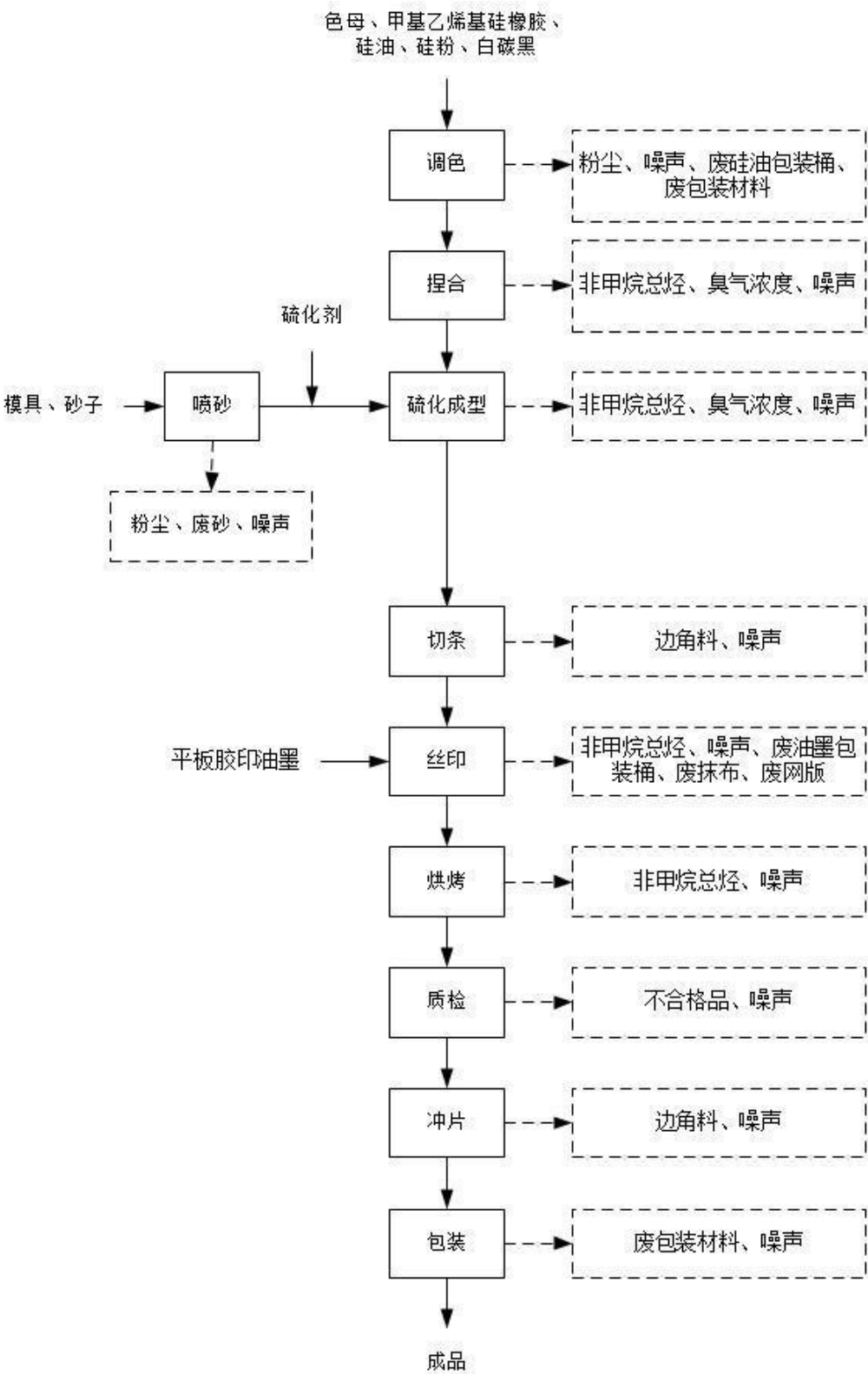
图 2 工艺流程图
