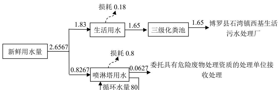
图 2-1 项目水平衡图 单位 t/d
