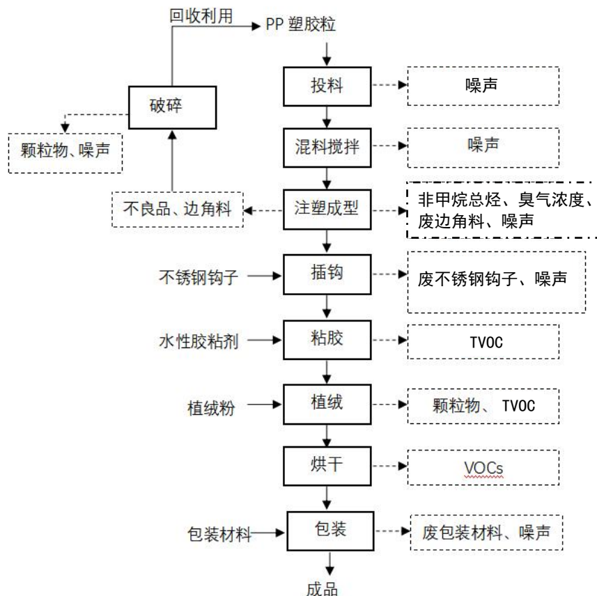
图 2.6-3 植绒衣架生产工艺流程及产污节点图
