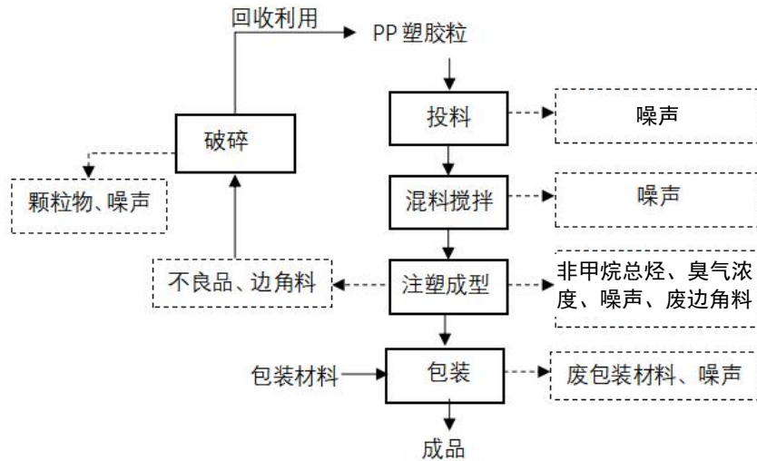
图 2.6-1 塑胶盒生产工艺流程及产污节点图
