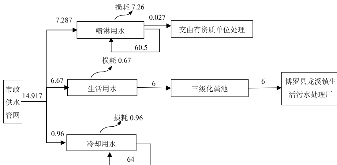
图 2.4-1 项目水平衡图 t/d
