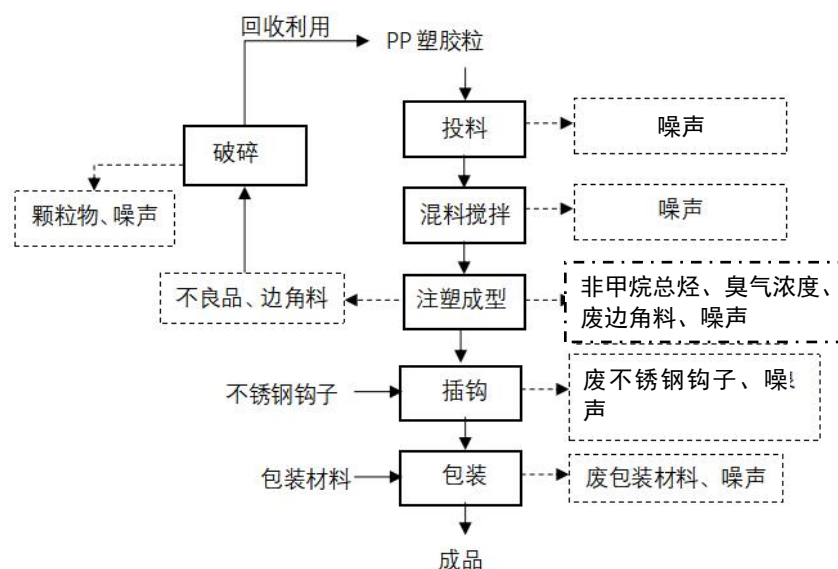
图 2.6-2 塑料衣架生产工艺流程及产污节点图
