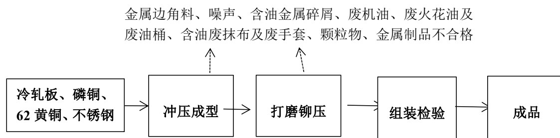
图 2-3 金属制品生产工艺流程图
