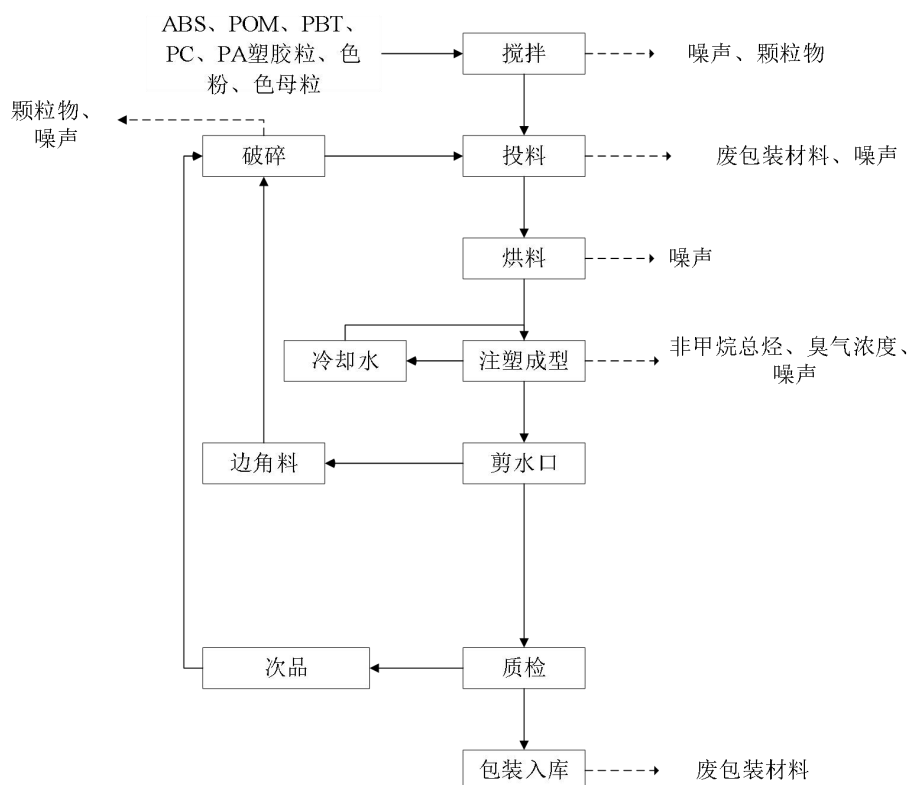
图 2-2 塑料制品生产工艺流程图
