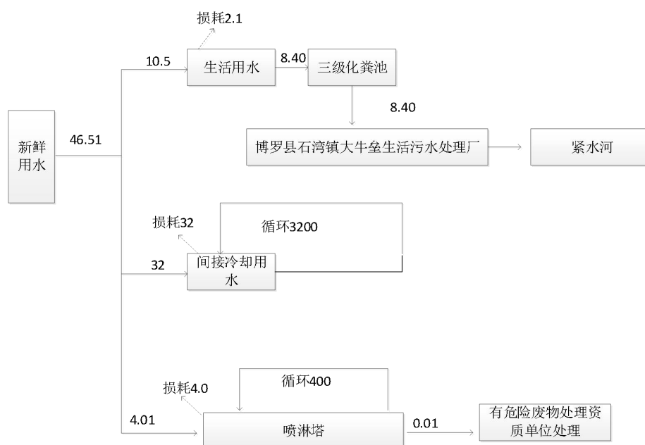
图 2-1 项目运营期水平衡图 (t/d)
