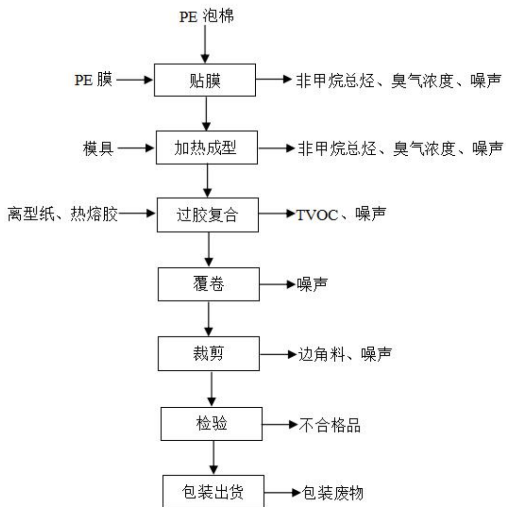
图 2-1 项目产品工艺流程
