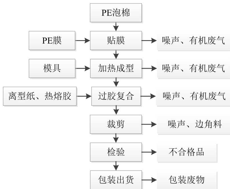
图 2-2 原项目生产工艺流程
