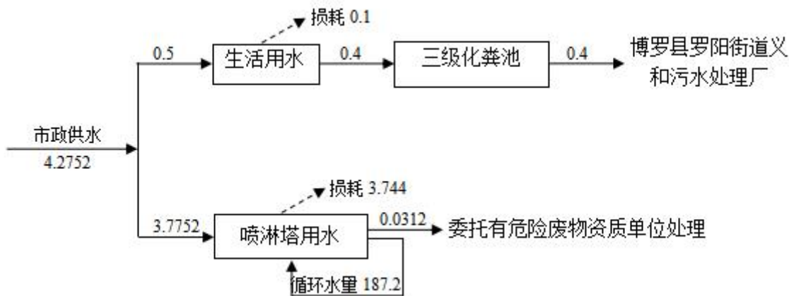
图 2-2 项目远期水平衡图 (t/d)
