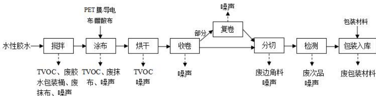
图 2-3 项目 PET 胶带、导电布胶带、醋酸布胶带生产工艺流程图
