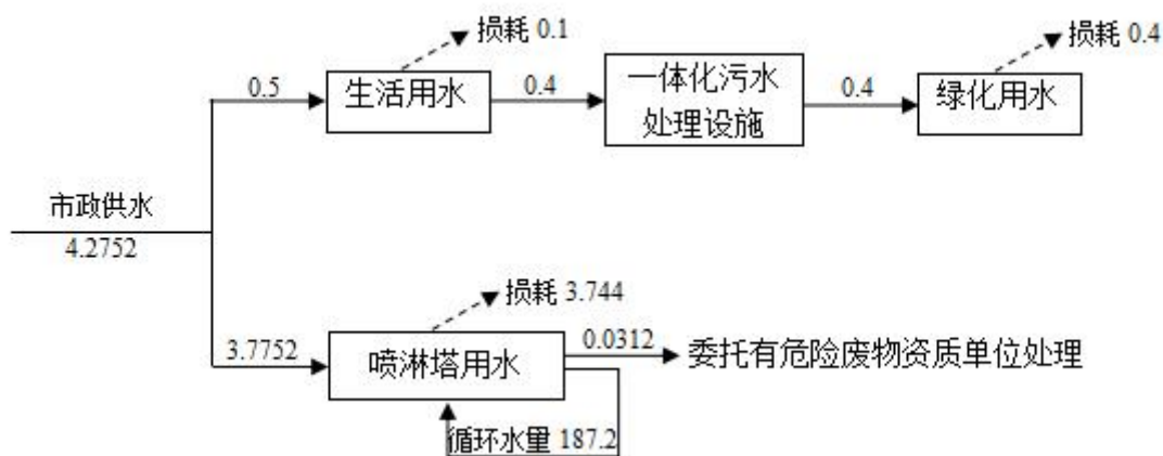
图 2-1 项目近期水平衡图（t/d）
